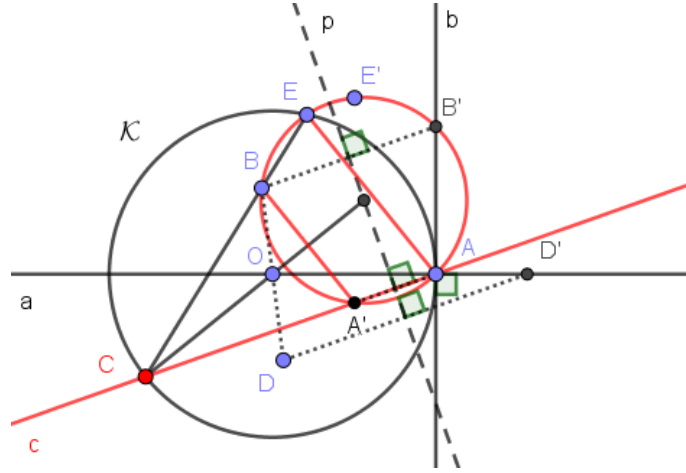
Slika 90: Stranski produkti Scimemijeve konstrukcije točke P (označeno z rdečo).
