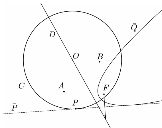
Slika 93: Konstrukcija dotikališča skupne tangente s krožnico. Vzeto iz [36, str. 40].
