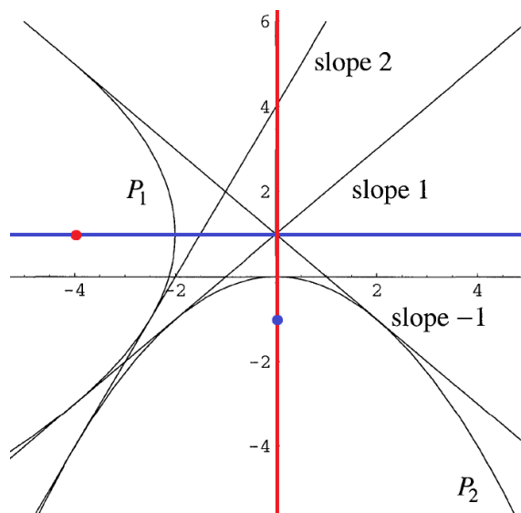
Slika 83: Konstrukcija skupnih tangent na paraboli. Preurejeno iz [7, str. 22].
