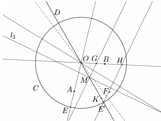
Slika 95: Nishimurijeva origami konstrukcija gorišča F (korak 13). Vzeto iz [36, str. 42].
