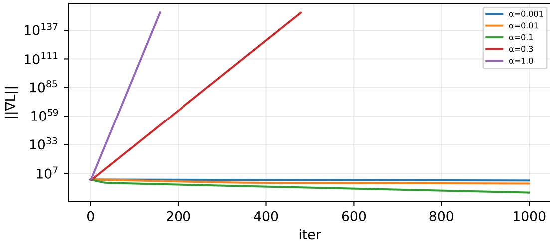
Gradient norm
