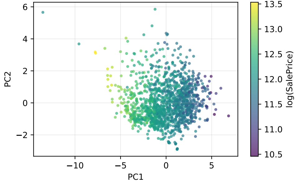
PCA projection
