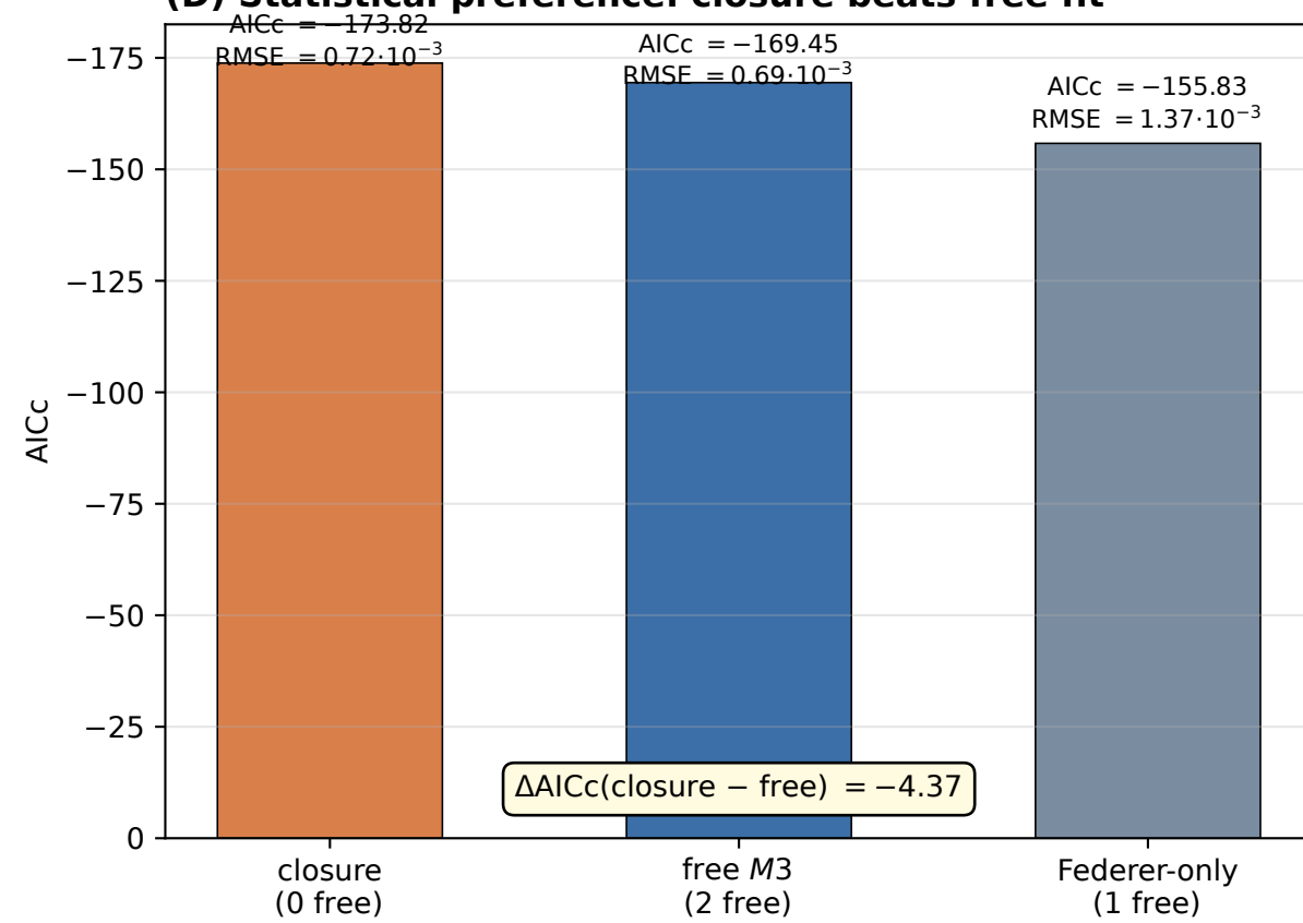
(D) Statistical preference: closure beats free fit
