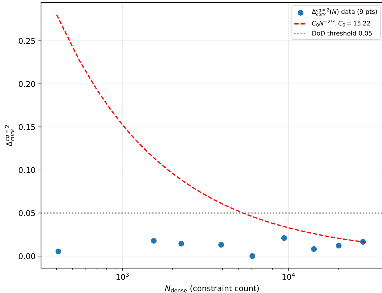
Pfad 2: 9-Punkt-A2-Bound (v5) C_0=15.22 , alle Werte unter Bound
