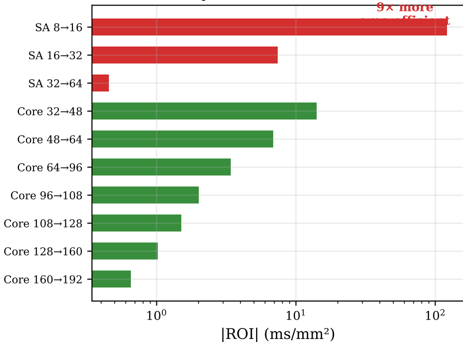
Area Efficiency: SA Dim vs Core Count (Prefill)
