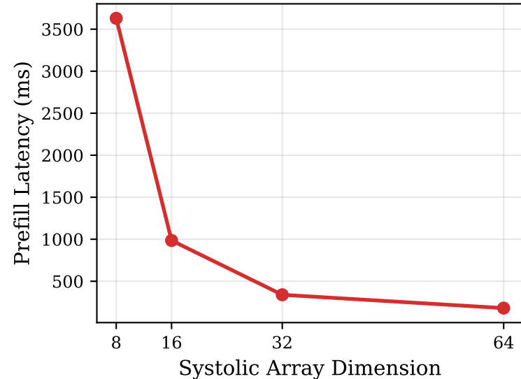
(a) SA Dim \rightarrow Prefill (Quadratic scaling)
