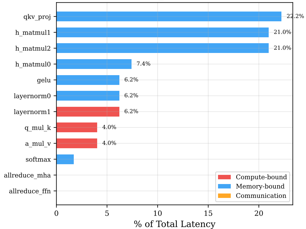
(b) llama_70b — Decode
