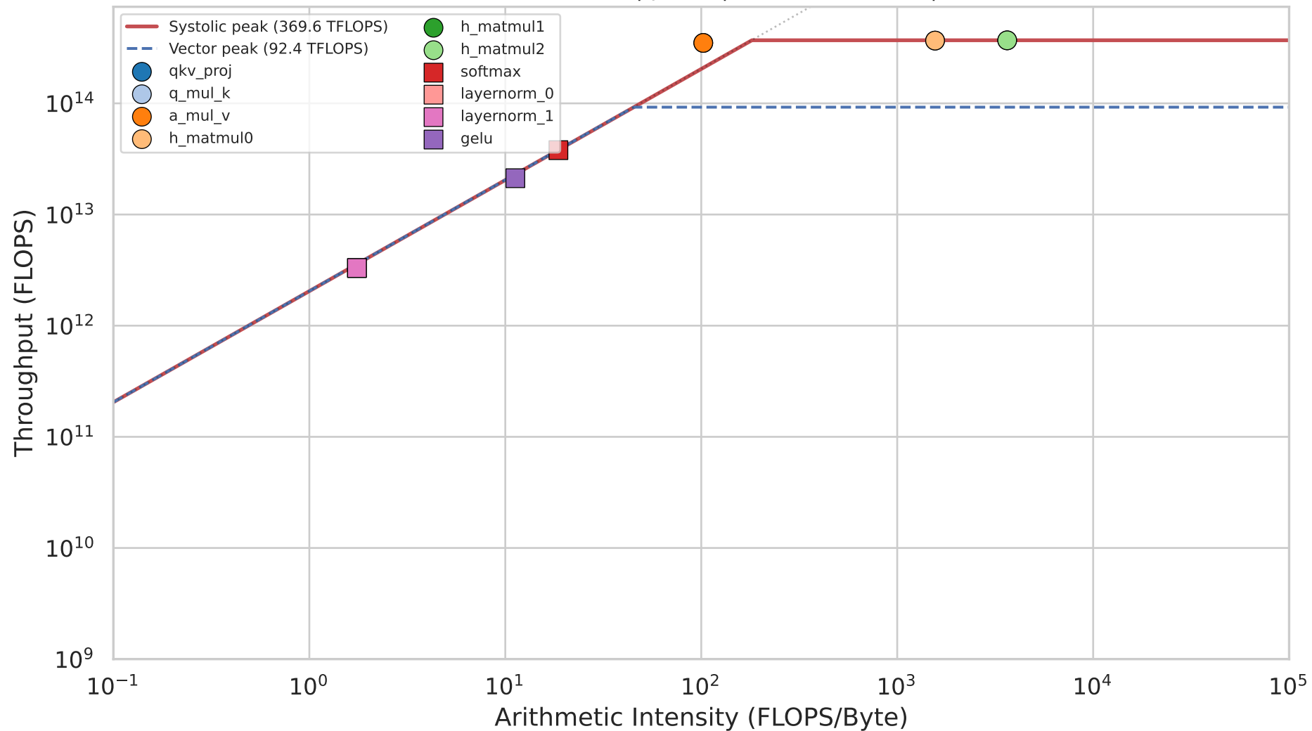
Roofline — LLaMA-70B | prefill | BS=32 SL=1024 | 4x GPU
