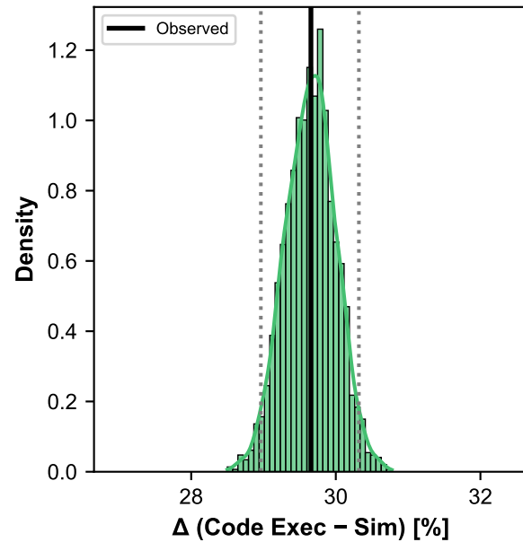
(C) \Delta = +29.66\% [28.96, 30.32]
