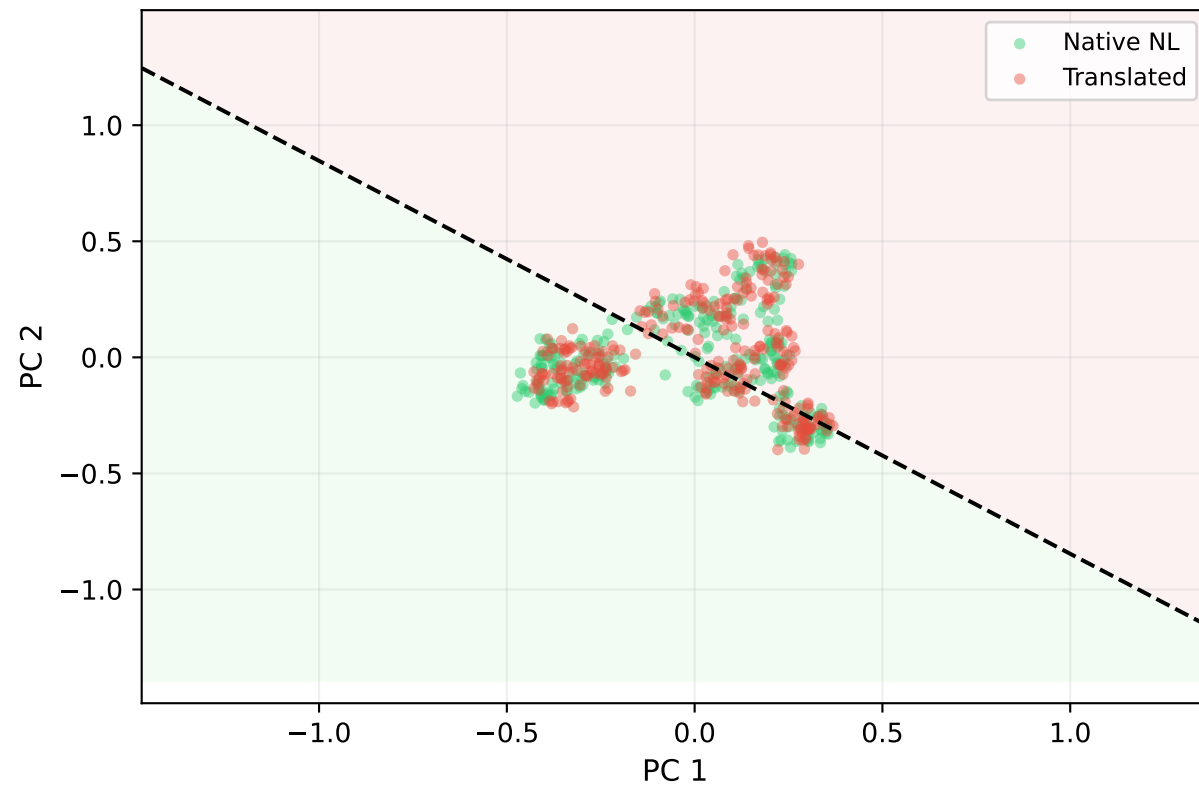
GPT-4o Acc=94.8% AUC=0.987
