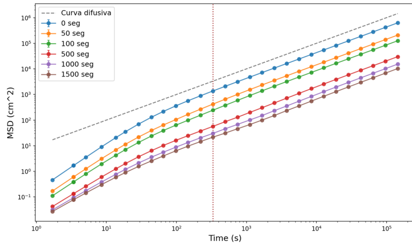
Figura 2.5: MSD para el segundo modelo, con tiempo constante de reposo.
