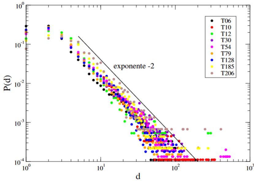
Figura 2.2: Distribución de desplazamientos cada 15 minutos para las tortugas en su hábitat natural.
