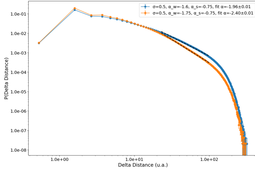
Figura 2.7: Distribución de desplazamientos a 15 minutos para \sigma_\theta = 0,5 , \alpha_S = 0,75 y \alpha_W = 1,6 y 1,75 .
