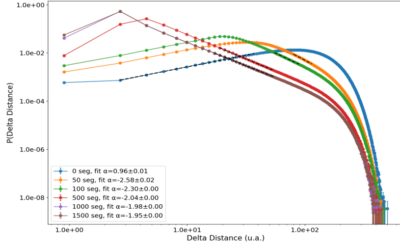
Figura 2.4: Distribución de desplazamiento para el segundo modelo, con tiempo constante de reposo.
