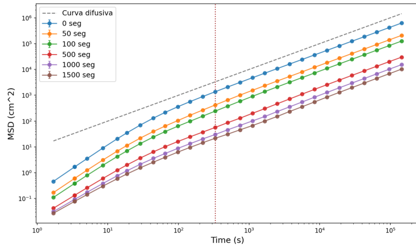
Figura 2.5: MSD para el segundo modelo, con tiempo constante de reposo.
