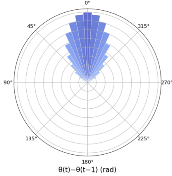
Figura 2.1: Esquema de un caminante aleatorio correlacionado. En cada paso, el individuo cambia su dirección de movimiento en un ángulo \eta_i sorteado de una distribución gaussiana de media nula y desviación estándar \sigma_\theta .
