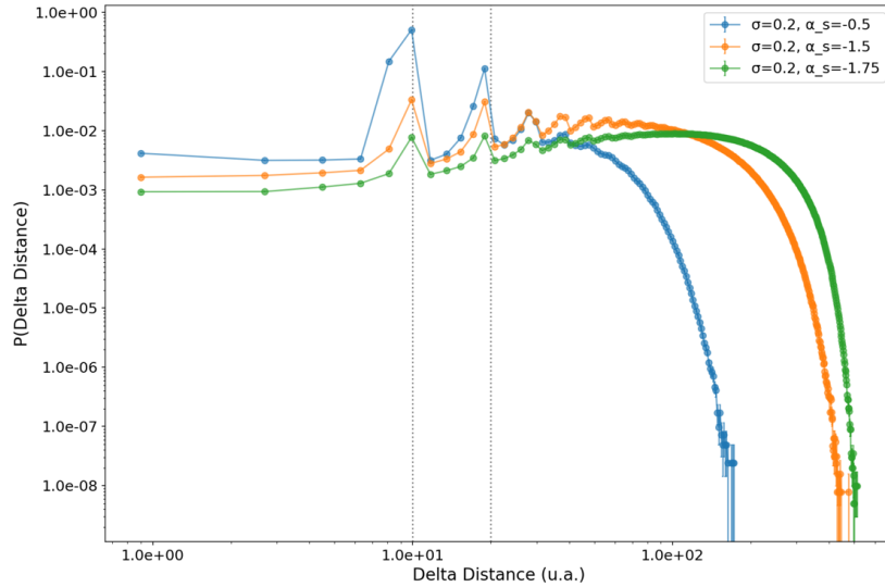
Figura 2.3: Distribución de desplazamiento para el primer modelo, con tiempo constante de caminata.
