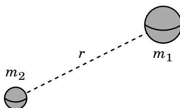
Obrázek 18: Two Body Problem
