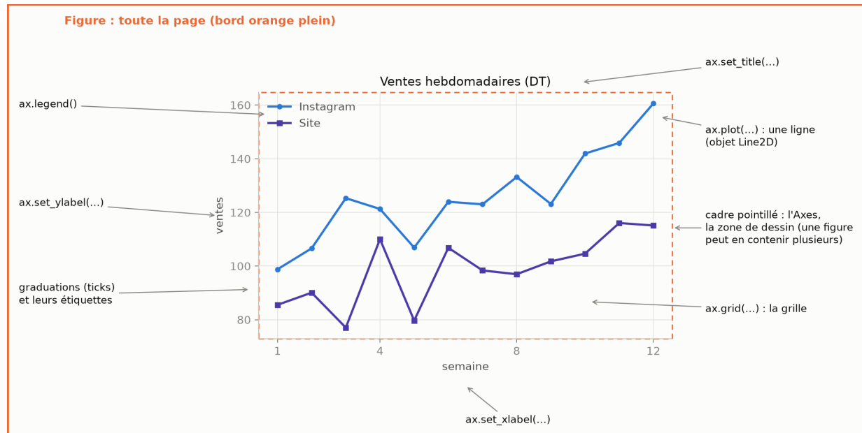
Figure 24: Les pièces d'un graphique matplotlib : la Figure (la page entière), l'Axes (le repère, cadre pointillé), puis les éléments dessinés dedans.
