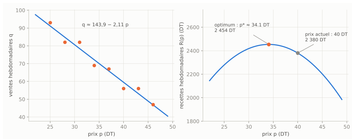
Figure 9: À gauche : les huit mesures et la droite de demande ajustée. À droite : les recettes prévues selon le prix, avec leur maximum vers 34 DT.
