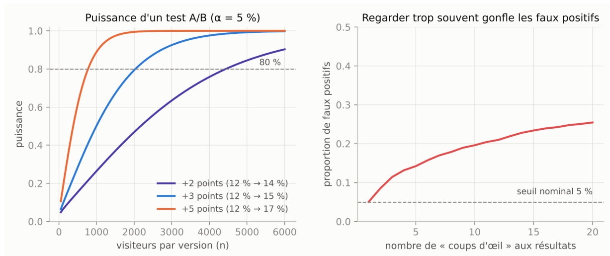
Figure 22:    gauche : puissance d'un test A/B en fonction du nombre de visiteurs, pour trois tailles d'effet.    droite : si l'on « jette un   il » aux r  sultats de plus en plus souvent et que l'on s'arr  te d  s que p < 0,05 , le taux de faux positifs explose (sous H_0 ).
