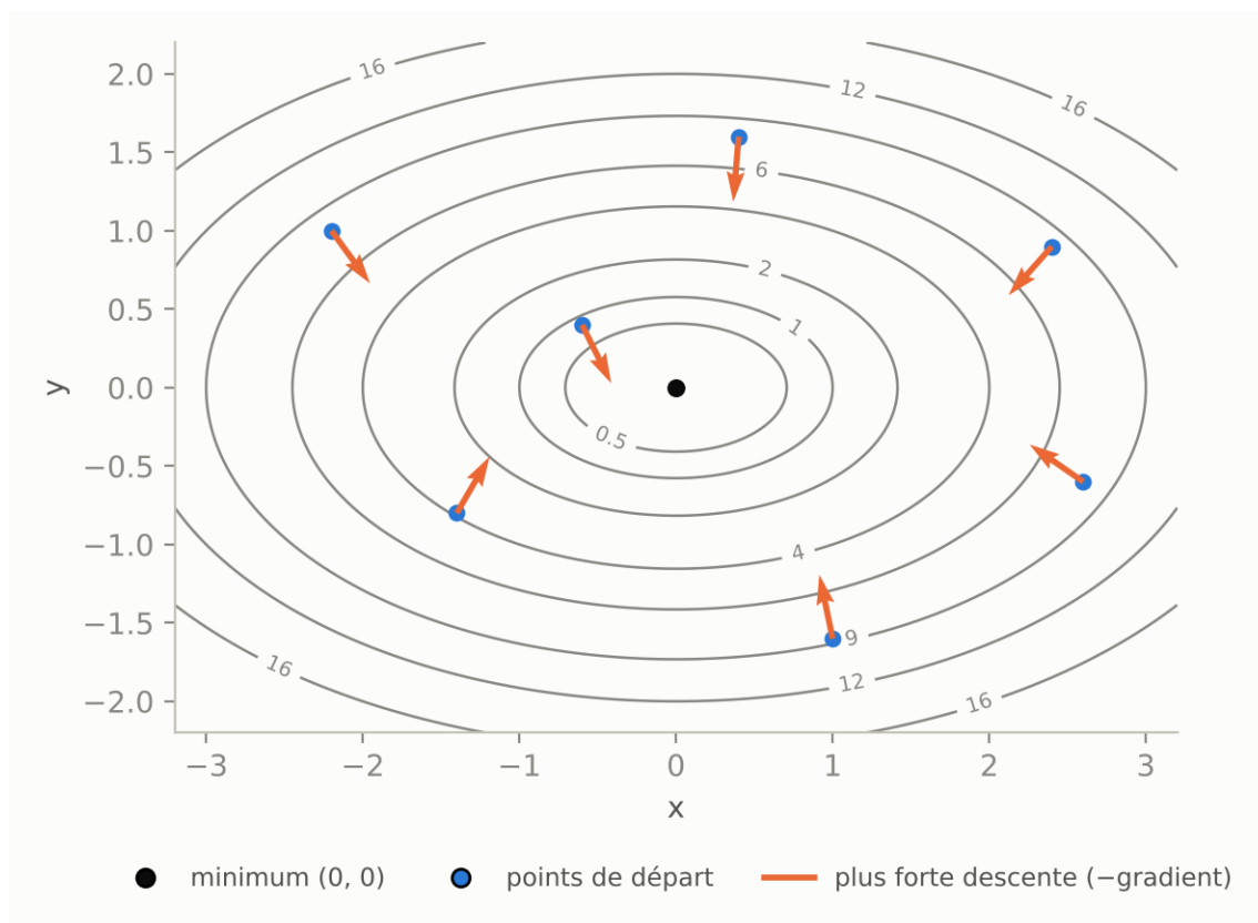
Figure 5: Courbes de niveau de f(x,y) = x^2 + 3y^2 (chaque ellipse est une « altitude » constante) et, en chaque point, la direction de la plus forte descente (−gradient). Les flèches sont perpendiculaires aux courbes de niveau et pointent vers le fond du bol.
