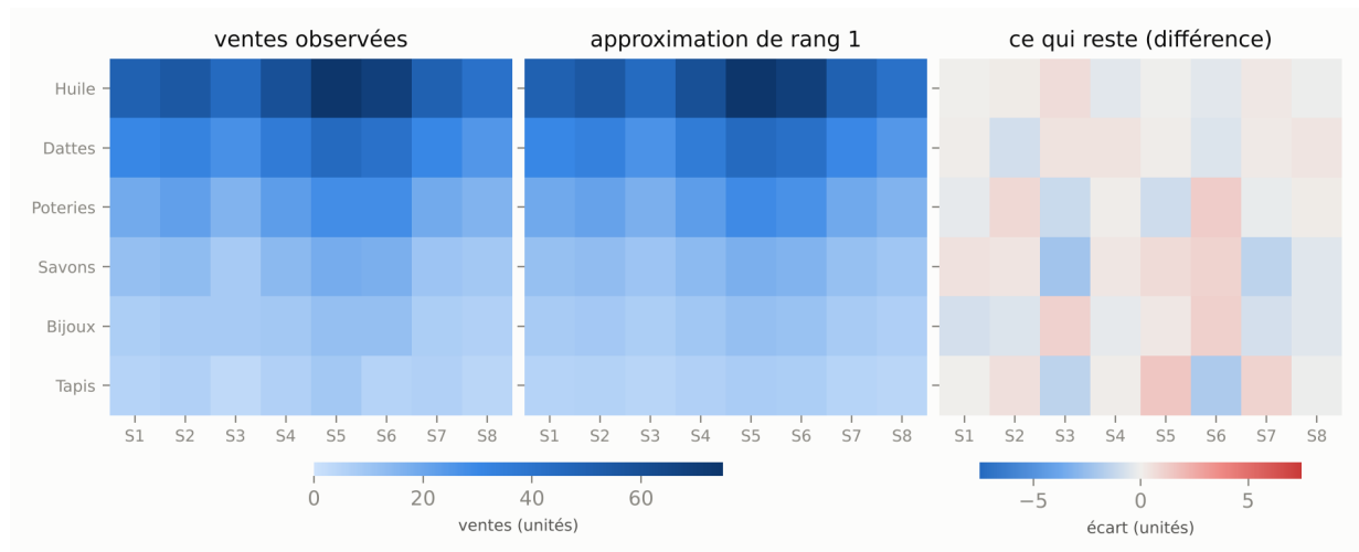
Figure 3: Ventés observées (à gauche), approximation par une seule couche (au centre) et ce qui reste (à droite). L'échelle de couleur est la même pour les deux premiers panneaux.
