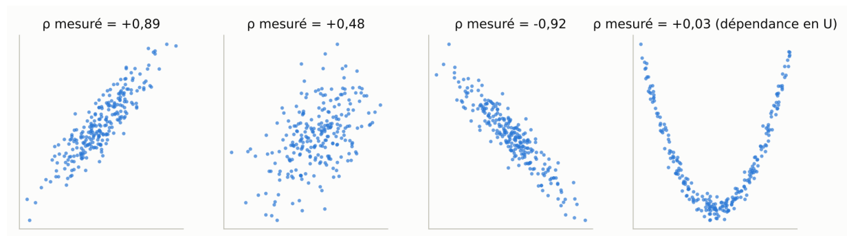
Figure 13: Quatre nuages de points et leur corrélation. Le dernier montre qu'une corrélation nulle n'implique pas l'indépendance.
