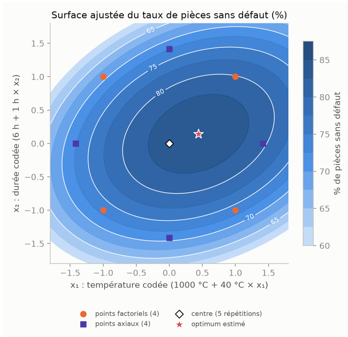
Figure 89: Surface ajustée du taux de pièces sans défaut en fonction de la température et de la durée (unités codées), avec les 13 points du plan composite centré et l'optimum estimé. Les courbes de niveau sont des ellipses allongées et inclinées autour du sommet.
