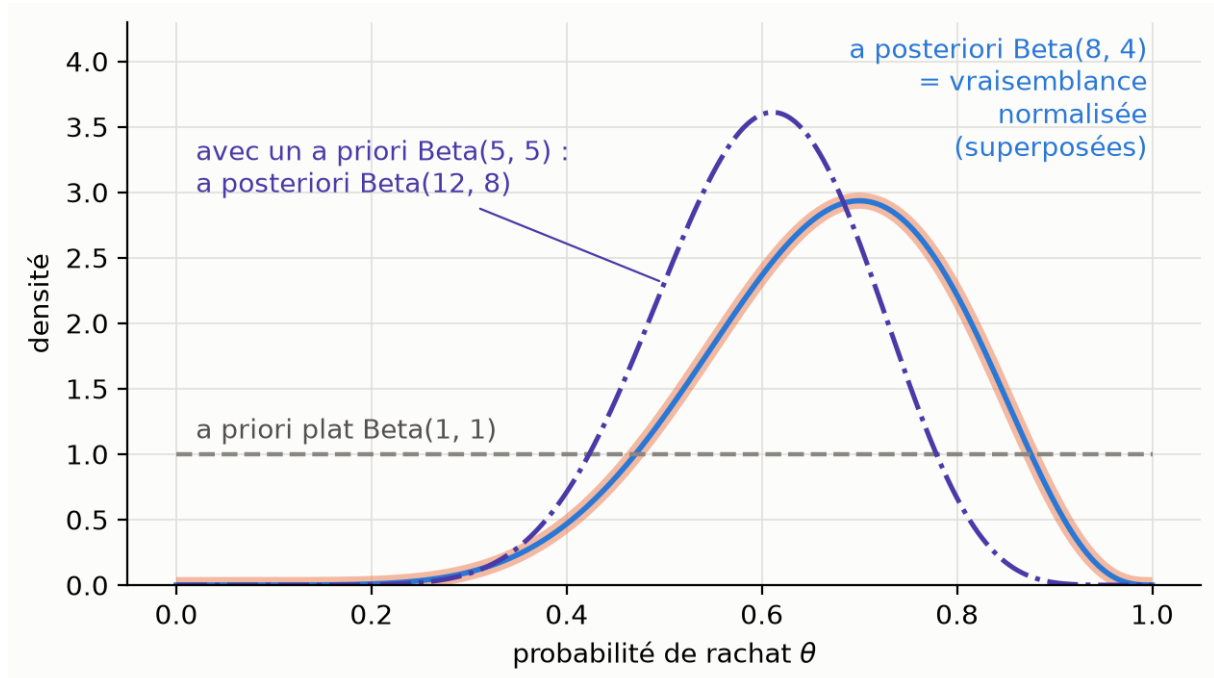
Figure 61: Avec 7 rachats sur 10 : l'a priori plat (tirets gris), la vraisemblance normalisée (orange épais) et l'a posteriori Beta(8, 4) (bleu) sont superposés ; avec un a priori informatif Beta(5, 5), l'a posteriori Beta(12, 8) (violet, tirets-points) est tiré vers 0,5.
