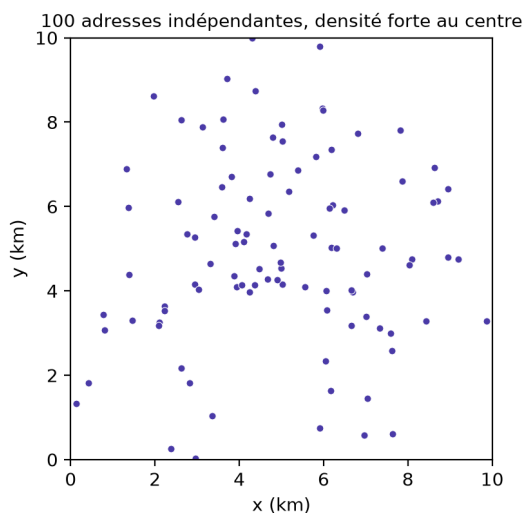
Figure 100: À gauche : 100 adresses indépendantes les unes des autres, mais avec une densité qui décroît du centre vers les bords. À droite : la fonction L(r) - r sort de l'enveloppe du hasard complet, alors qu'il n'y a aucune interaction entre les points.
