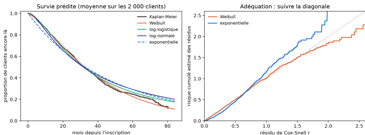
Figure 59: À gauche : survie de Kaplan-Meier des 2 000 clients et survie moyenne prédite par quatre modèles paramétriques. À droite : résidus de Cox-Snell du modèle de Weibull et du modèle exponentiel avec covariables ; le bon modèle suit la diagonale.
