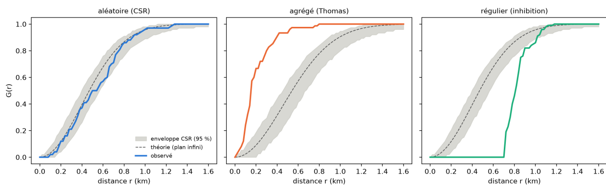
Figure 98: Fonction G (part des points dont le plus proche voisin est à moins de r ) pour les trois semis, avec l'enveloppe de Monte-Carlo (bandeau gris, 499 semis CSR de même taille) et la courbe théorique du plan infini (pointillés).
