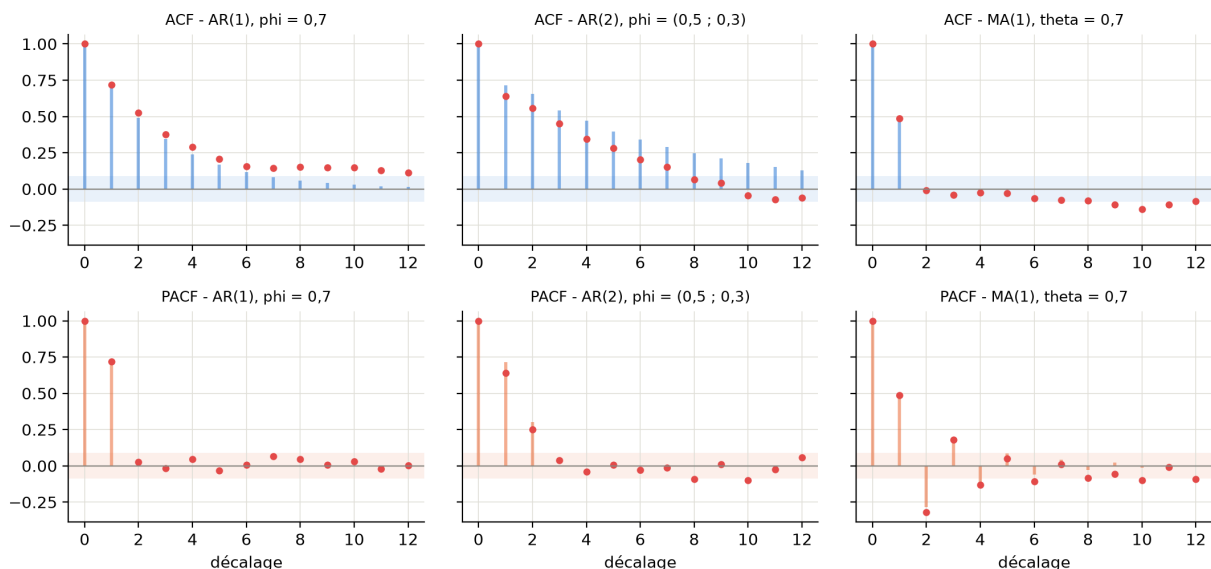
Figure 41: Signatures théoriques (barres) et empiriques (points rouges, 500 observations simulées) : l' AR(1) a une ACF qui décroît et une PACF qui s'arrête au décalage 1 ; l' AR(2) a une PACF qui s'arrête au décalage 2 ; le MA(1) a une ACF qui s'arrête au décalage 1 et une PACF qui décroît.
