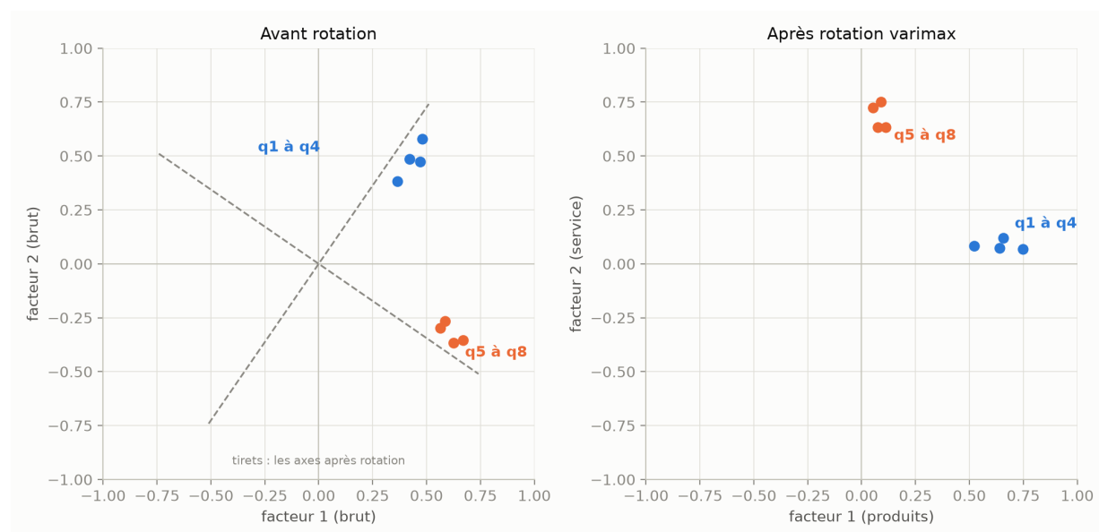
Figure 27: Les huit questions dans le plan des deux facteurs : avant rotation (à gauche) et après rotation varimax (à droite). La rotation fait tourner les axes sans modifier la position relative des points ; après rotation, chaque question est proche d'un seul axe.
