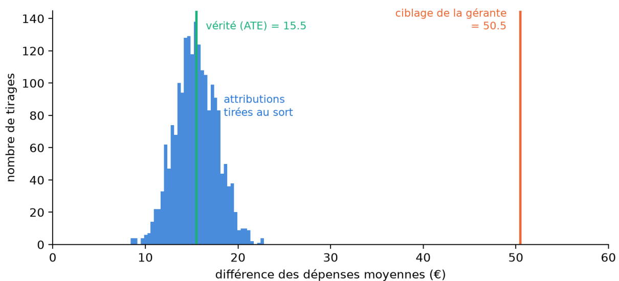
Figure 70: Distribution de la différence naïve quand l'attribution est tirée au sort (2 000 tirages), comparée à la valeur obtenue avec le ciblage de la gérante et à la vérité.
