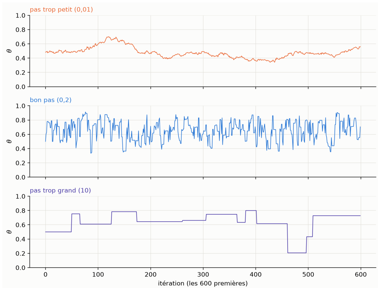
Figure 63: Trois traces de la marche aléatoire de Metropolis pour la loi Beta(8, 4), avec trois pas différents. Pas trop petit : la chaîne rampe lentement. Bon pas : la chaîne explore toute la zone de forte densité. Pas trop grand : la chaîne reste longtemps bloquée sur des paliers.
