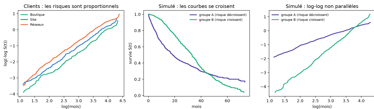
Figure 57: À gauche : graphique log-log des trois canaux de la boutique (courbes presque parallèles). Au centre et à droite : deux groupes simulés dont les risques se croisent (courbes de survie qui se coupent, courbes log-log non parallèles).
