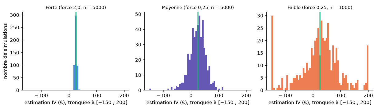
Figure 80: Distribution de l'estimateur IV sur 500 répétitions, pour un instrument fort, moyen et faible. La ligne verte marque la vraie valeur (25 €). Plus l'instrument est faible, plus la distribution est étalée et plus elle comporte de valeurs aberrantes.
