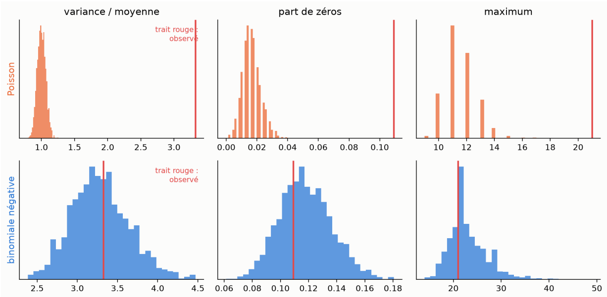
Figure 66: Vérification prédictive a posteriori de deux modèles pour le nombre de commandes annuelles des clients du canal Boutique. En haut, le modèle de Poisson : les histogrammes des trois statistiques répliquées (variance sur moyenne, part de zéros, maximum) sont loin de la valeur observée (trait rouge). En bas, la binomiale négative : la valeur observée est au milieu des répliques.
