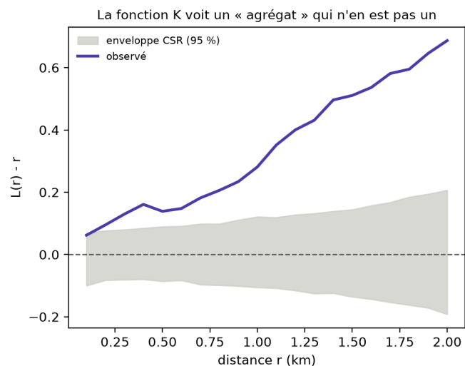
Figure 100: À gauche : 100 adresses indépendantes les unes des autres, mais avec une densité qui décroît du centre vers les bords. À droite : la fonction L(r) - r sort de l'enveloppe du hasard complet, alors qu'il n'y a aucune interaction entre les points.
