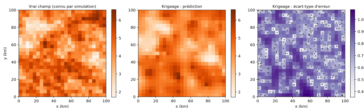
Figure 95: De gauche à droite : le vrai champ de délais (connu car simulé), la prédiction par krigage ordinaire à partir des 200 mesures, et l'écart-type d'erreur de krigage (les points noirs sont les 200 livraisons mesurées). L'incertitude est faible près des mesures et monte dans les zones qui en sont éloignées.
