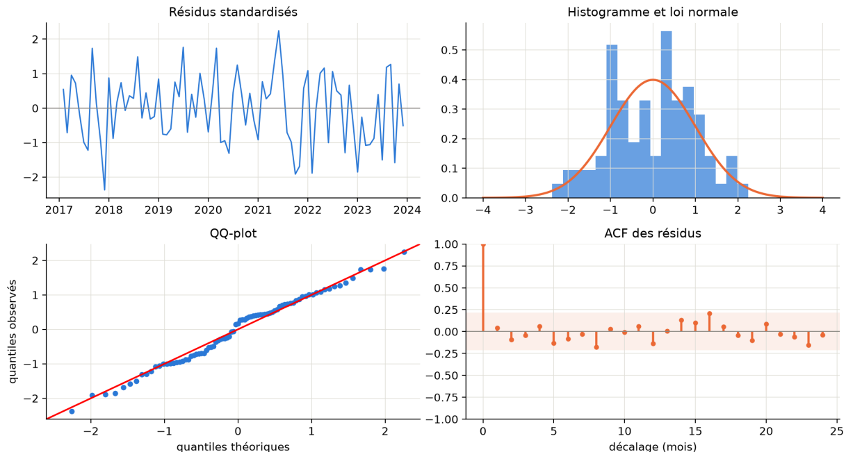
Figure 43: Diagnostic des résidus du SARIMAX(1,1,1)(0,1,1) 12 : résidus standardisés sans structure, histogramme proche de la loi normale, QQ-plot proche de la droite, ACF sans barre hors bande.
