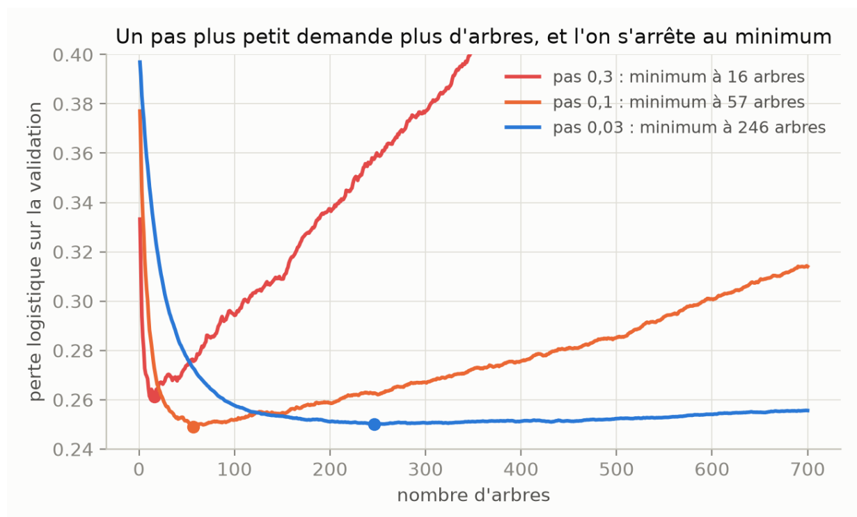
Figure 24: Perte logistique sur le jeu de validation selon le nombre d'arbres, pour trois pas d'apprentissage. Chaque courbe passe par un minimum puis remonte : le modèle se met à sur-apprendre. Plus le pas est petit, plus le minimum est atteint tard.
