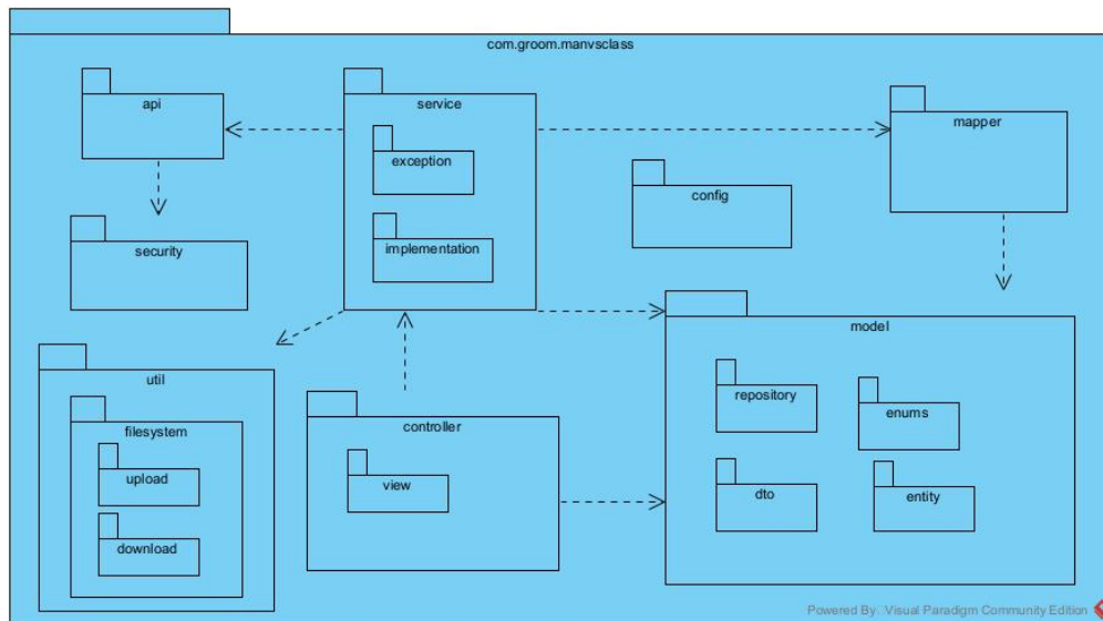
Figure 12: Diagramma dei Package
