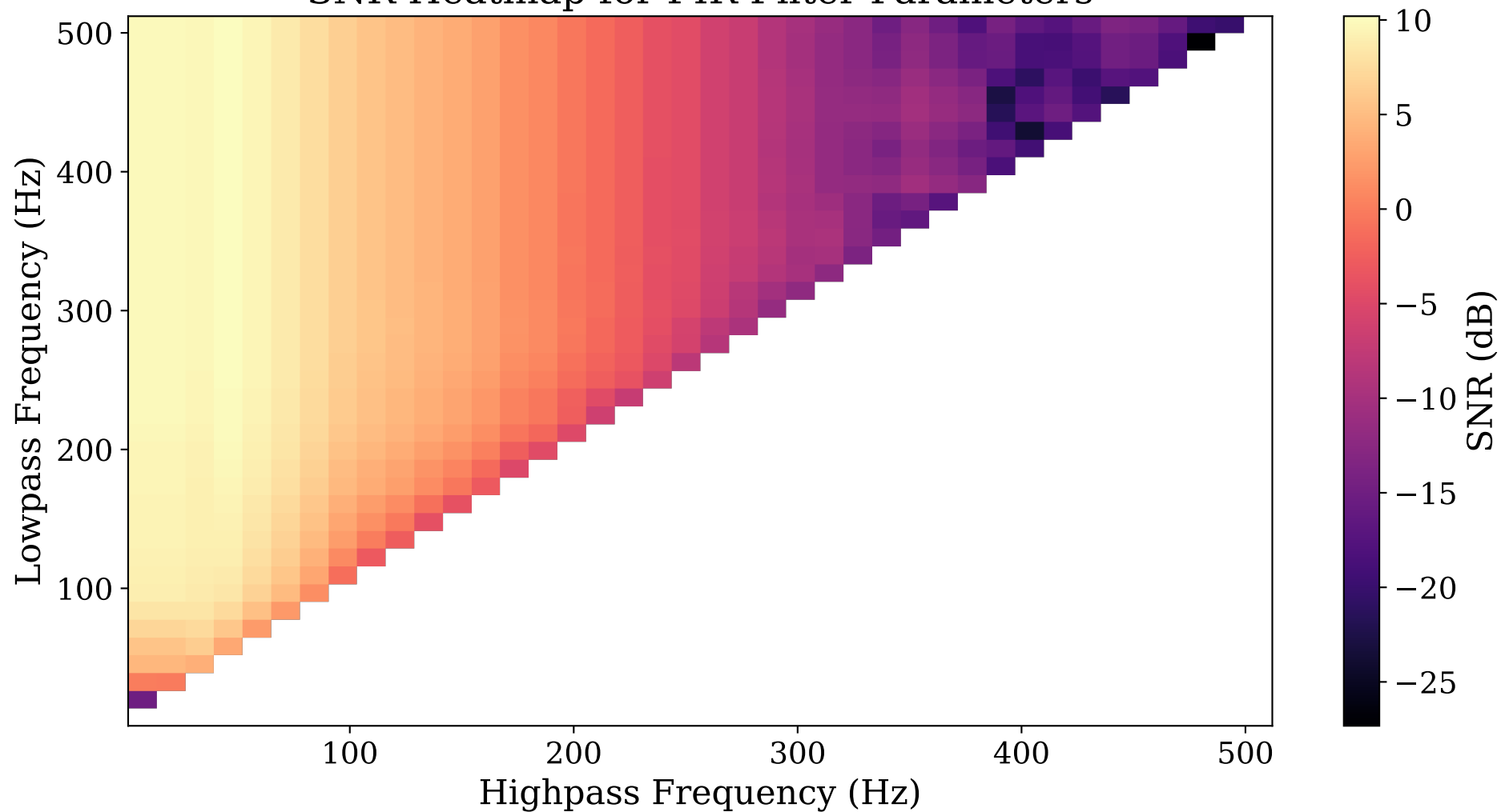
SNR Heatmap for FIR Filter Parameters
