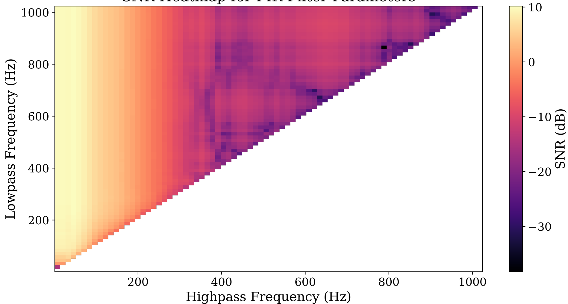
SNR Heatmap for FIR Filter Parameters
