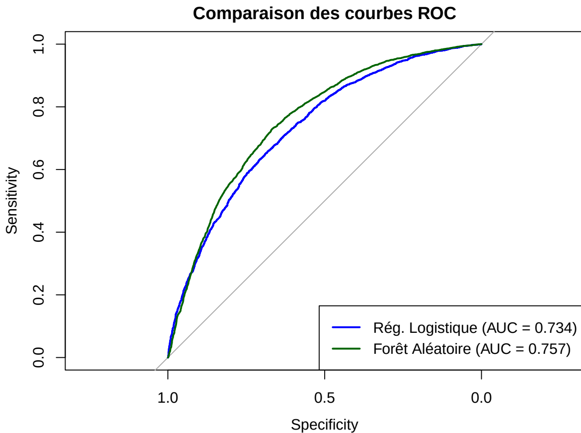
FIGURE 1 : Comparaison des courbes ROC
