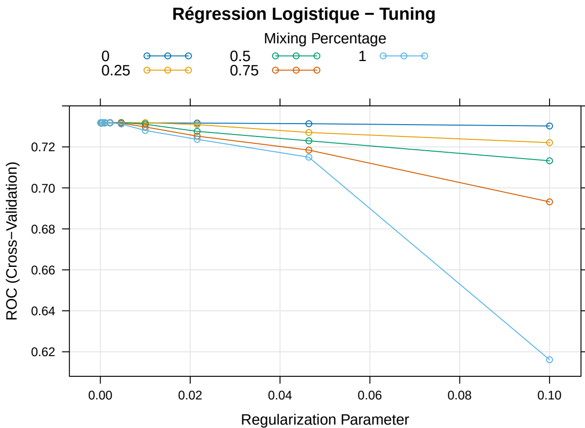
FIGURE 1 : Performance de la régression logistique selon les hyperparamètres
