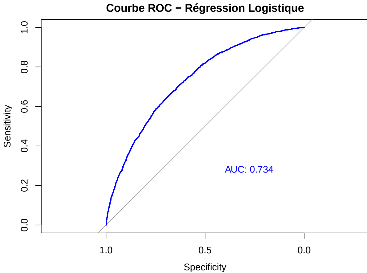
FIGURE 2 : Courbe ROC – Régression Logistique
