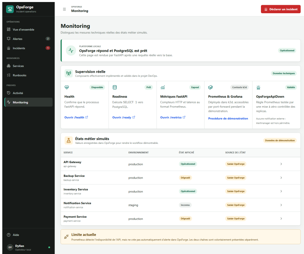
Figure 5 — La page Monitoring sépare la « Supervision réelle » (health, readiness, métriques, Prometheus/Grafana, règle testée) des « États métier simulés » (source : saisie OpsForge), et affiche la limite : les alertes Prometheus ne sont pas ingérées dans OpsForge.
