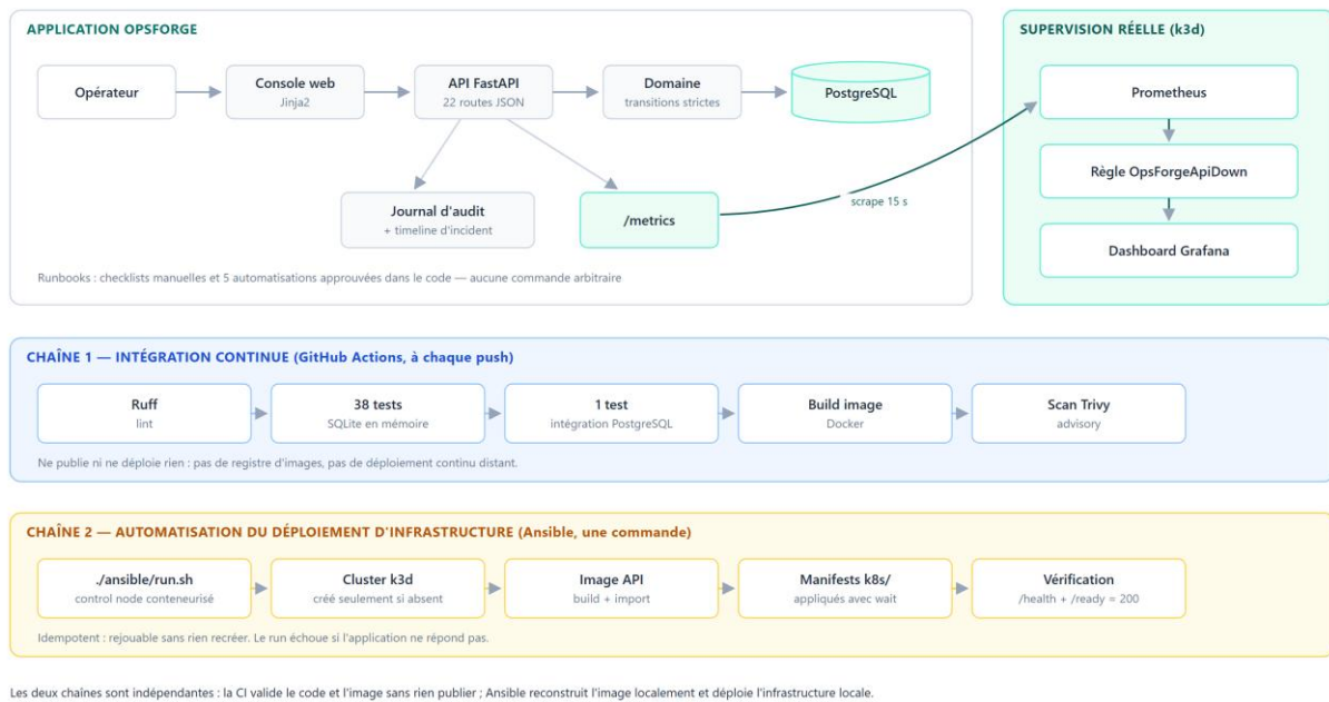
Figure 2 — Architecture logique : l'application et sa supervision réelle (haut), puis les deux chaînes d'outillage (bas). La CI valide le code et l'image sans rien publier ; Ansible reconstruit l'image localement et déploie l'infrastructure.
