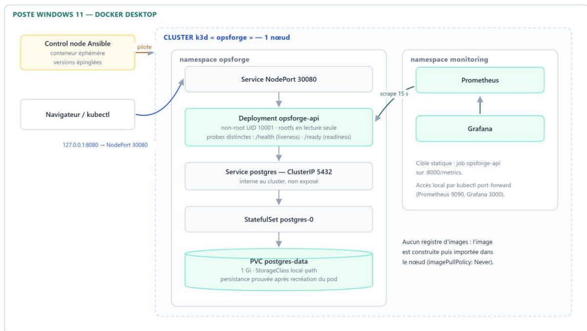
Figure 3 — Topologie déployée : tout tient sur un poste Windows 11 avec Docker Desktop. Le control node Ansible est un conteneur éphémère qui pilote le cluster k3d ; l'API est exposée sur 127.0.0.1:8080 via le NodePort 30080.
