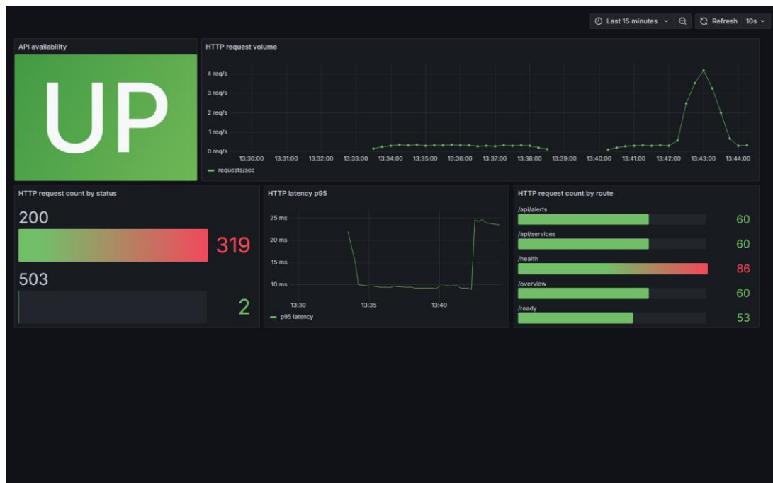
Figure 8 — Le dashboard « OpsForge Monitoring » pendant la session de preuve : disponibilité UP, volume de requêtes (le creux correspond à la panne provoquée), 319 réponses 200 et 2 réponses 503 au redémarrage, latence p95 et répartition par route.
