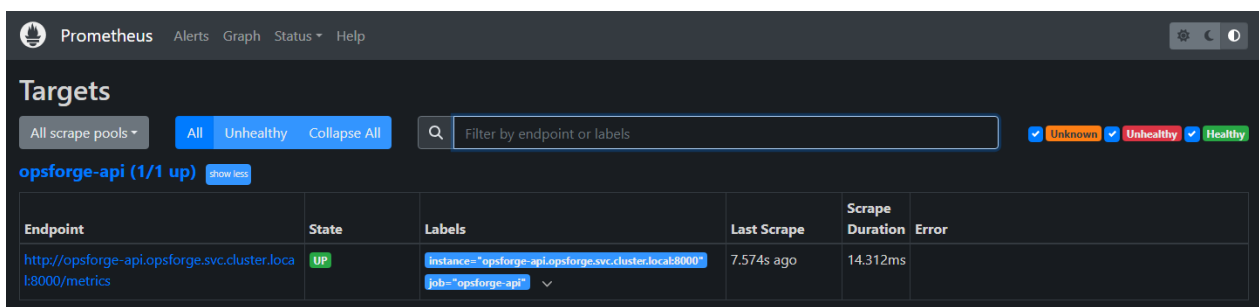
Figure 6 — Prometheus scrape réellement l'API : la cible opsforge-api (1/1 up) pointe sur /metrics du Service Kubernetes, état UP.
