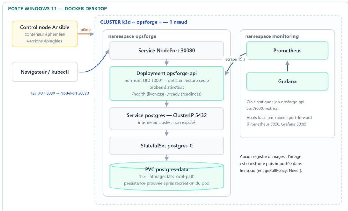
Figure 3 — Topologie déployée : tout tient sur un poste Windows 11 avec Docker Desktop. Le control node Ansible est un conteneur éphémère qui pilote le cluster k3d ; l'API est exposée sur 127.0.0.1:8080 via le NodePort 30080.
