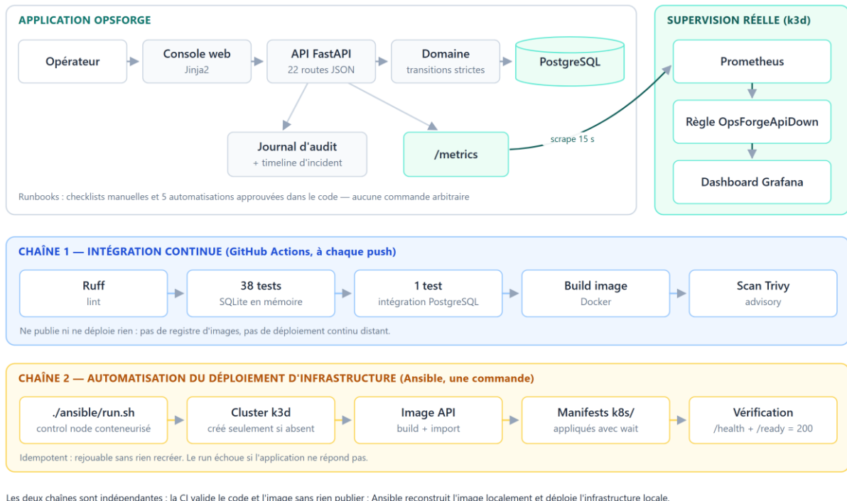
Figure 2 — Architecture logique : l'application et sa supervision réelle (haut), puis les deux chaînes d'outillage (bas). La CI valide le code et l'image sans rien publier ; Ansible reconstruit l'image localement et déploie l'infrastructure.
