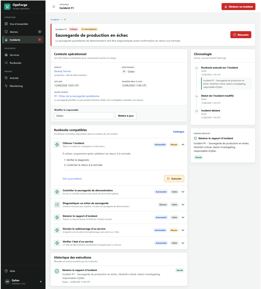
Figure 5 — Le Command Center d'un incident : contexte opérationnel, alerte source, runbooks compatibles (manuel ou automatisé, niveau de risque), chronologie issue du journal d'audit et historique des exécutions.
