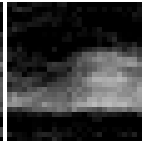
HyperLISTA
