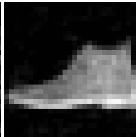
LISTA
