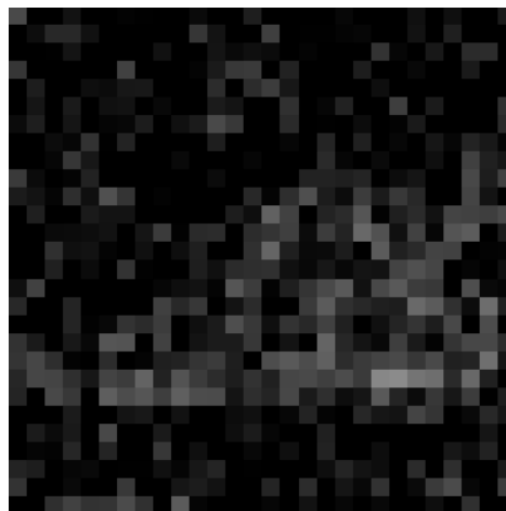
ISTA
