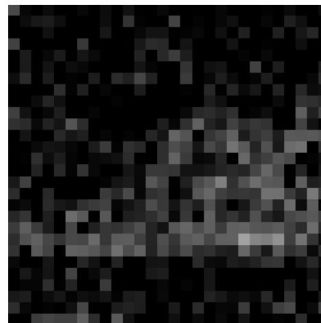
FISTA
