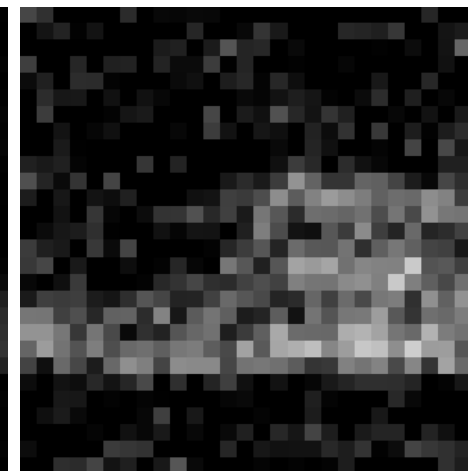
ALISTA
