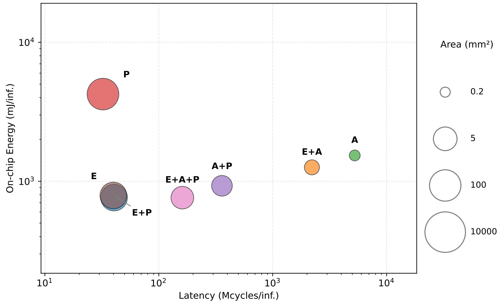
vs. SAURIA — VGG-16 FP16
