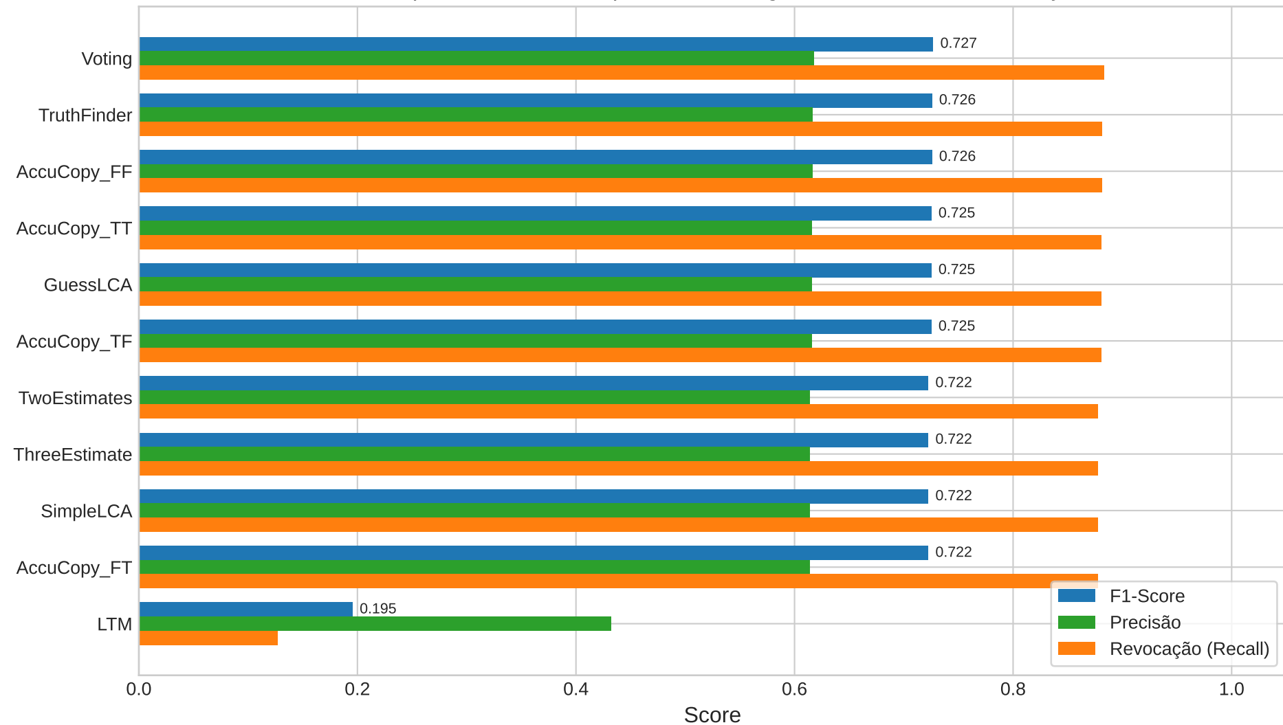
Comparativo de Desempenho entre Algoritmos de Truth Discovery
