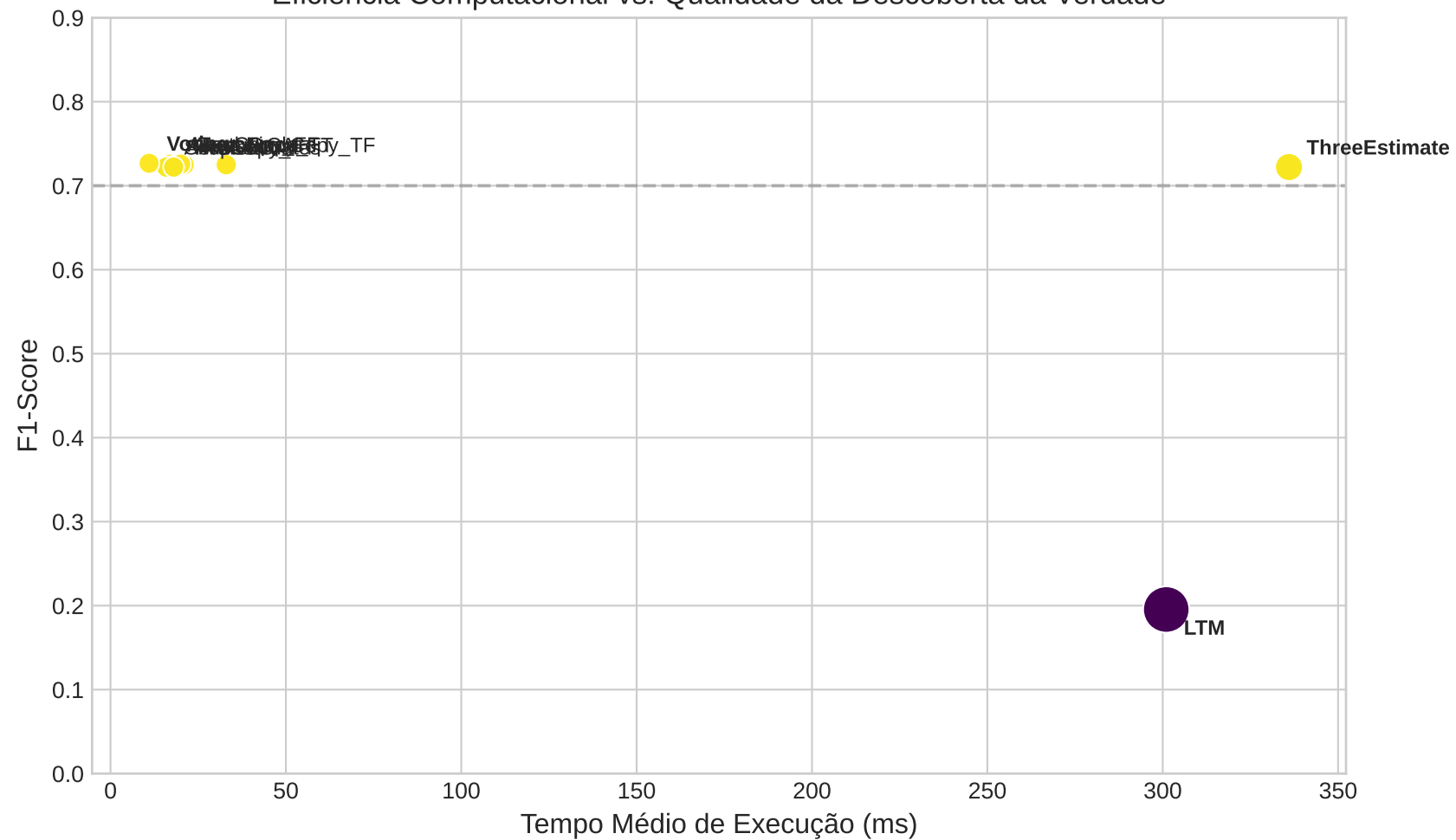
Eficiência Computacional vs. Qualidade da Descoberta da Verdade
