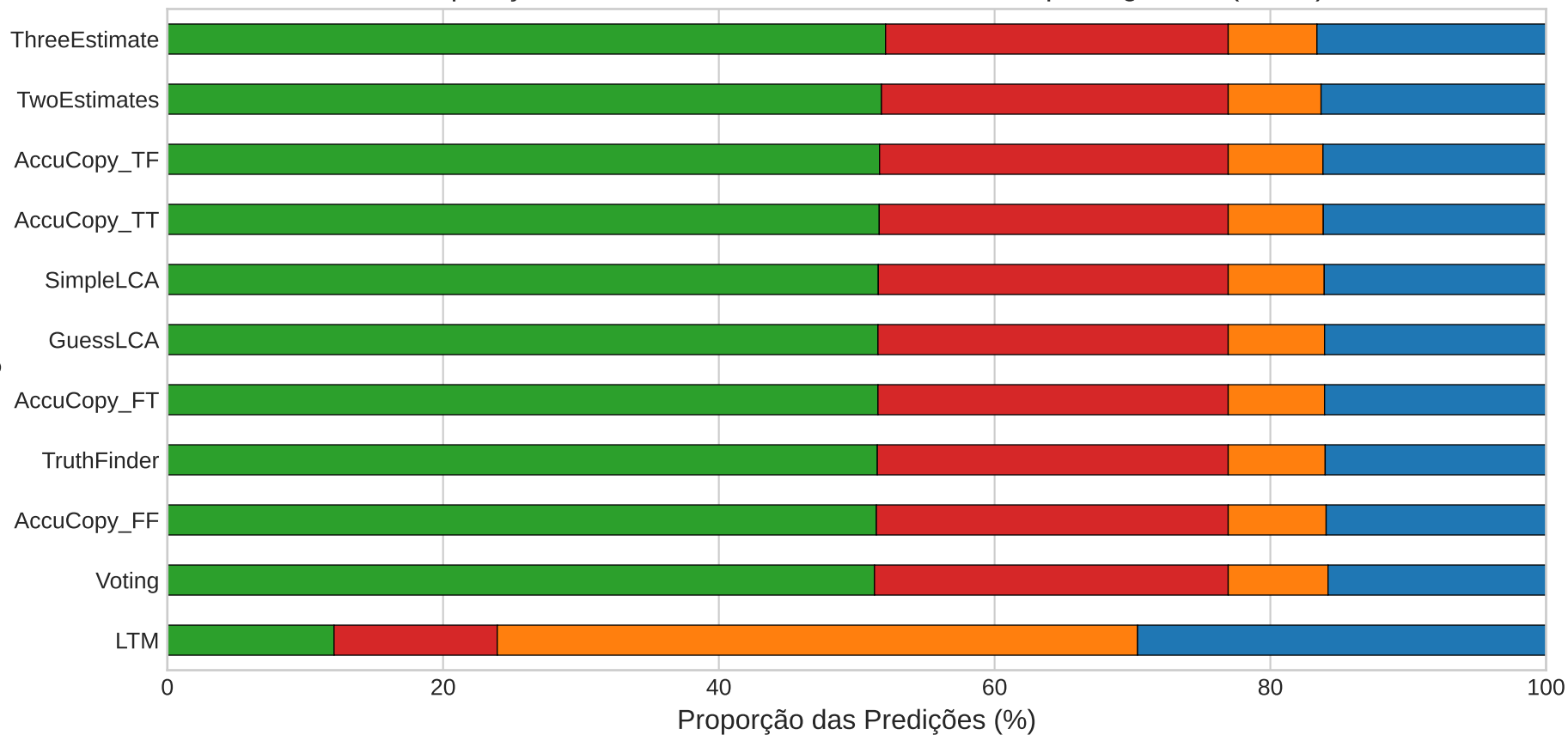
Composição da Matriz de Confusão Normalizada por Algoritmo (100%)
