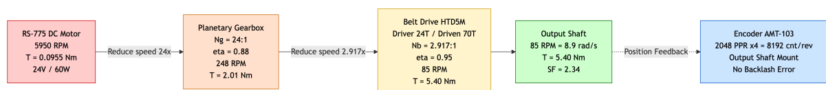
รูปที่ 3.2: แผนผังห่วงโซ่การส่งกำลังแสดงการเปลี่ยนแปลงความเร็วและแรงบิด ตั้งแต่มอเตอร์ถึงแขนกล พร้อมตำแหน่ง Encoder ที่ Output Shaft
