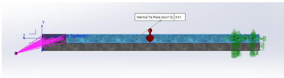
รูปที่ 3.14: โมเดลจำลอง FEA แสดงจุดจับยึด Fixture (สกรู) และทิศทางของภาระแรง Remote Load (ลูกศรสีแดง)
