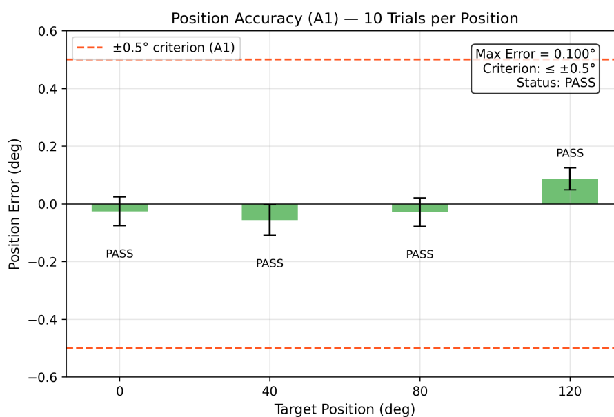
รูปที่ 5.4: ความแม่นยำตำแหน่ง (A1) ที่ทุก Workstation: Mean Error \pm\sigma เทียบกับเกณฑ์ \pm 0.5^\circ
