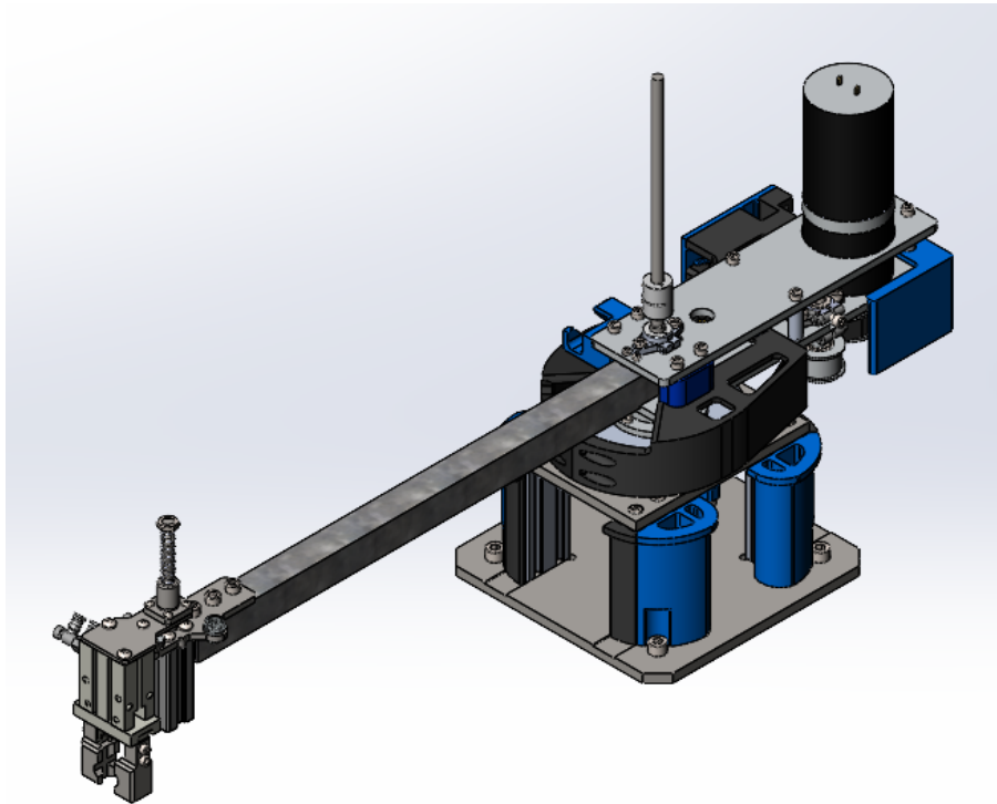
รูปที่ 3.4: CAD Assembly ของระบบเชิงกล แสดงส่วนประกอบหลักทั้งหมด
