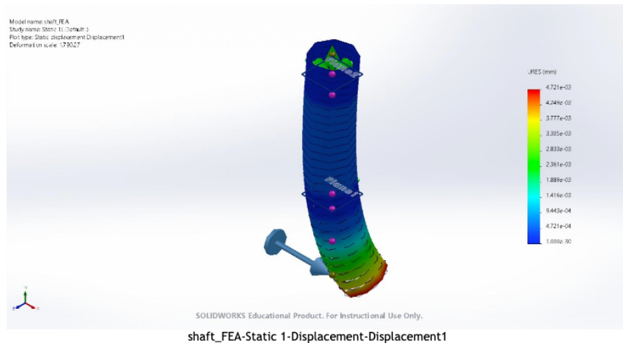
รูปที่ 3.8: ผล FEA เพลลา: ระยะการเบี่ยงเบน (URES Displacement) ( \text{Max} = 4.721 \times 10^{-3} \text{ mm} ที่ปลายเพลลา)
