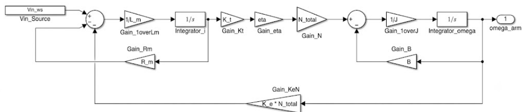
รูปที่ 3.26: Simulink Block Diagram ของแบบจำลอง DC Motor ที่ใช้ใน Grey-box Parameter Estimation แสดง Free Parameters ที่ปรับค่าโดย greyst
