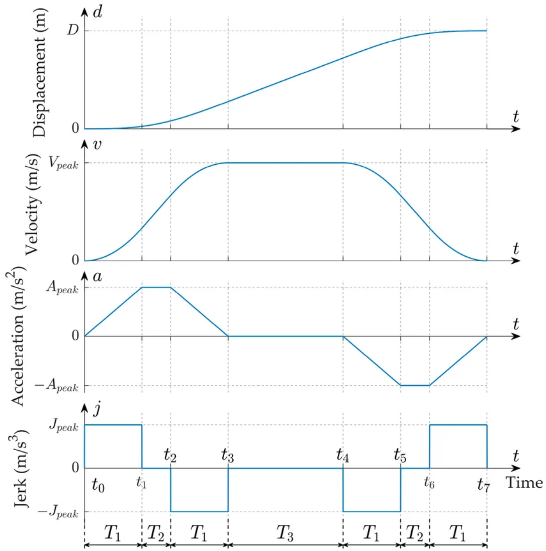
รูปที่ 2.7: โปรไฟล์การเคลื่อนที่แบบ S-Curve (Jerk-Limited) แสดงความสัมพันธ์เชิงจลนศาสตร์ทั้ง 7 เฟส
