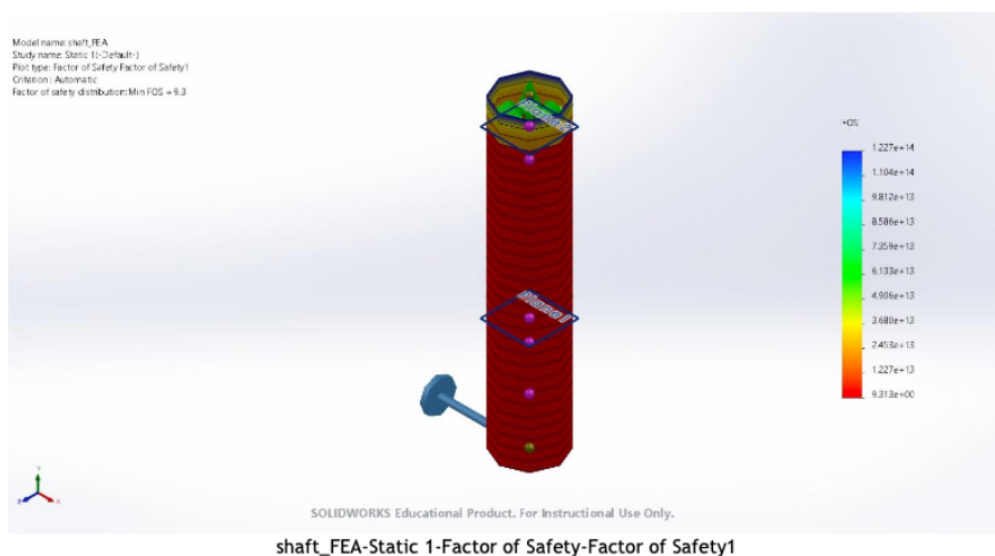
รูปที่ 3.9: ผล FEA เพลลา: ค่าความปลอดภัย (Factor of Safety) ( \text{Min FOS} = 9.313 บริเวณตำแหน่ง Belt Pulley)
