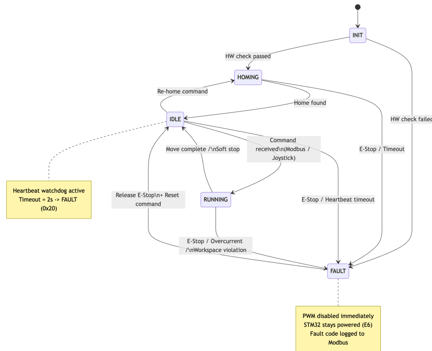
รูปที่ 4.11: แผนภาพสถานะการทำงานของระบบ (Application FSM) ของระบบควบคุม
