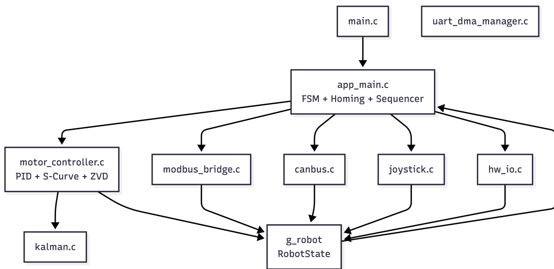
รูปที่ 4.12: สถาปัตยกรรมระบบ (Cyber-Physical System Architecture) ของหุ่นยนต์
