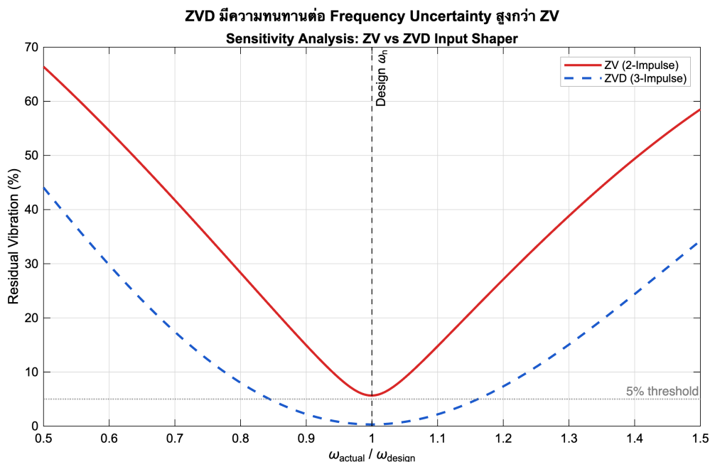
รูปที่ 3.38: Sensitivity Analysis เปรียบเทียบ ZV (สีแดง) และ ZVD (สีน้ำเงิน) แสดง Residual Vibration เมื่อ \omega_{actual} / \omega_{design} เบี่ยงจาก 1.0 ZVD รักษา Residual Vibration ต่ำกว่า 5% ในย่านกว้างกว่า ZV อย่างมีนัยสำคัญ
