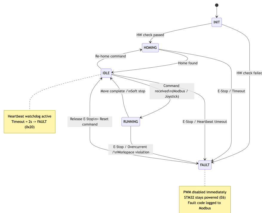
รูปที่ 4.11: แผนภาพสถานะการทำงานของระบบควบคุม (Application FSM) ของระบบควบคุม
