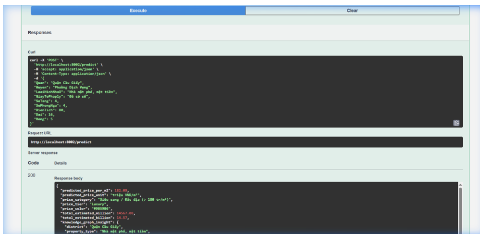
Hình 7.6 — Kết quả dự đoán giá nhà từ REST API (đơn vị: triệu VND/m 2 )
