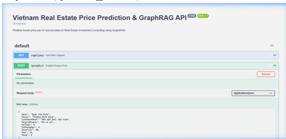
Hình 7.a — Giao diện API Swagger UI POST /predict (House Price) — Dữ liệu đặc trưng nhà
