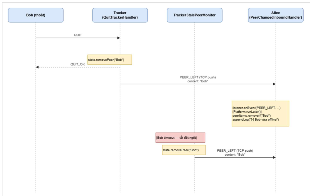
Hình 10. Luồng push PEER_LEFT khi peer rời mạng
