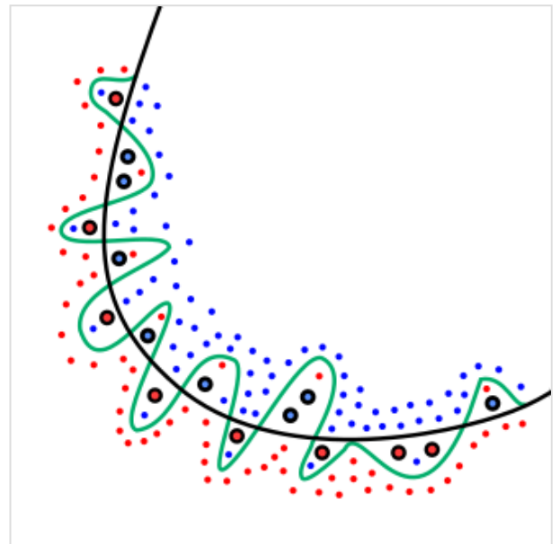
Hình 1. Đường màu xanh lục thể hiện mô hình quá khớp và đường màu đen thể hiện một mô hình chính quy. Trong khi đường xanh lục bám sát dữ liệu huấn luyện tốt nhất thì nó lại quá phụ thuộc vào dữ liệu và dường như sẽ có tỉ lệ lỗi cao trên các dữ liệu chưa biết đến (dữ liệu thử nghiệm) so với đường màu đen.
