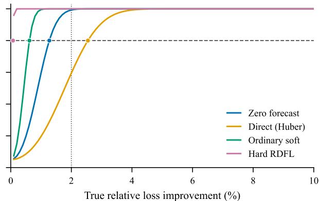
(d) Archived historical pipeline: equivalence test
