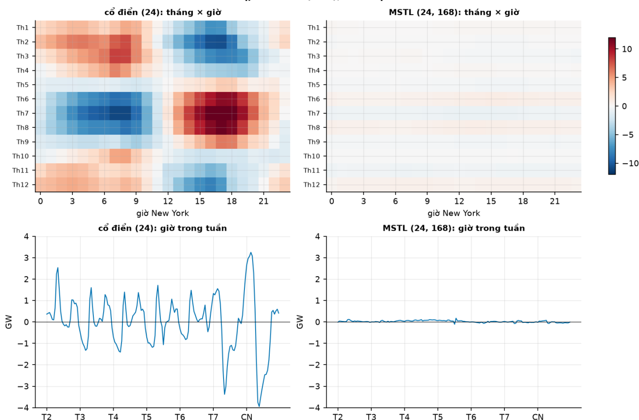
Trung bình phần dư (GW) — cổ điển còn mùa vụ ngày đối theo mùa (trên) và nhịp cuối tuần (dưới); MSTL sạch cả hai
