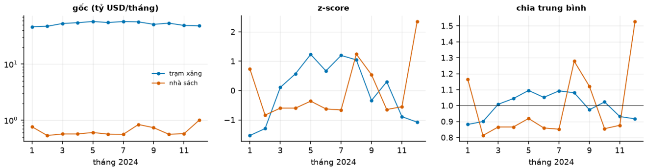
Hai chuỗi lệch nhau 80 lần: z-score xoá mất độ lớn dao động tương đối, chia trung bình giữ lại
