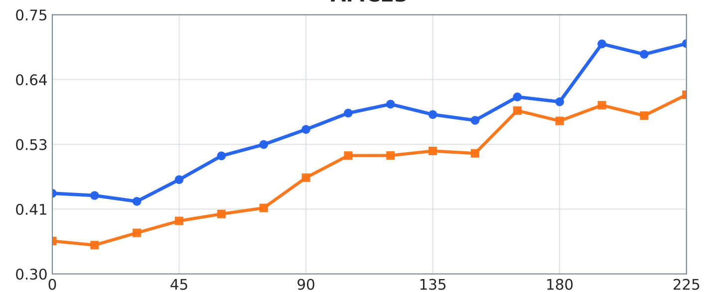
AMC23
