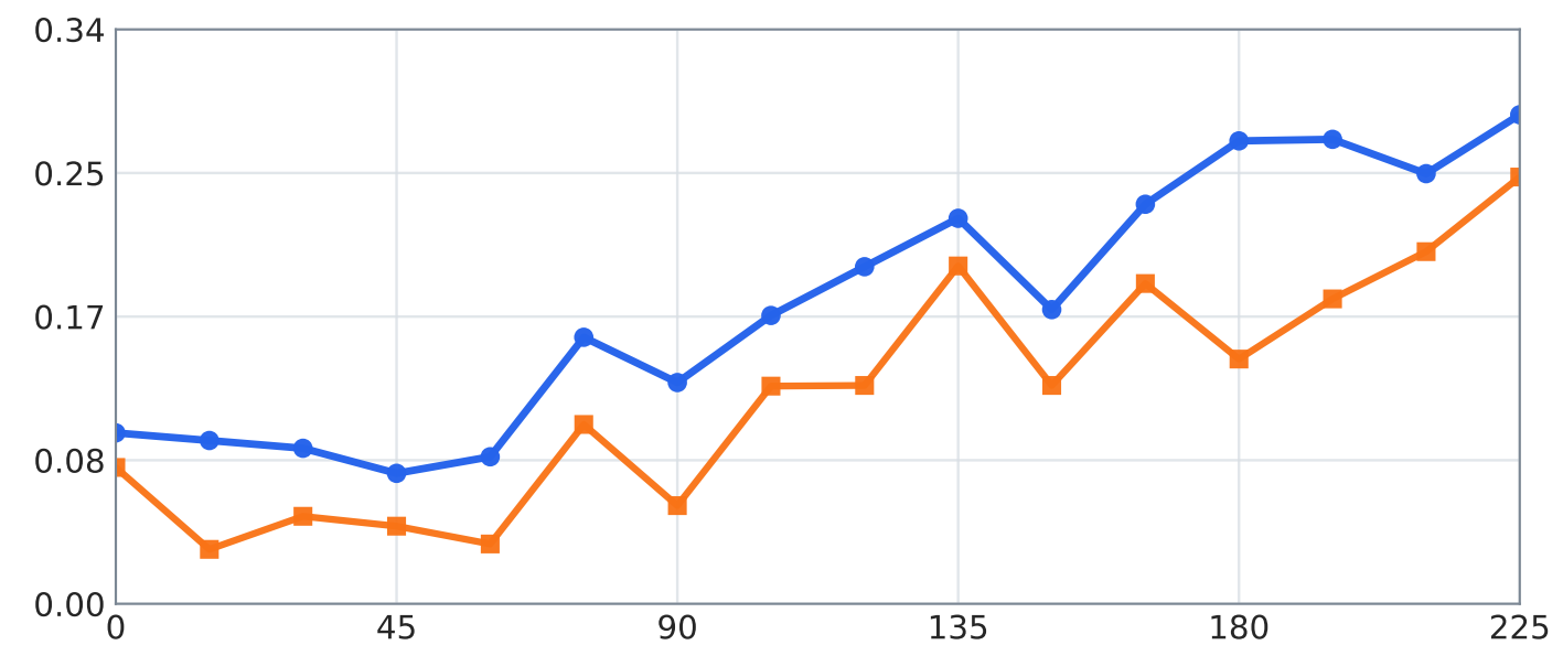
AIME24
