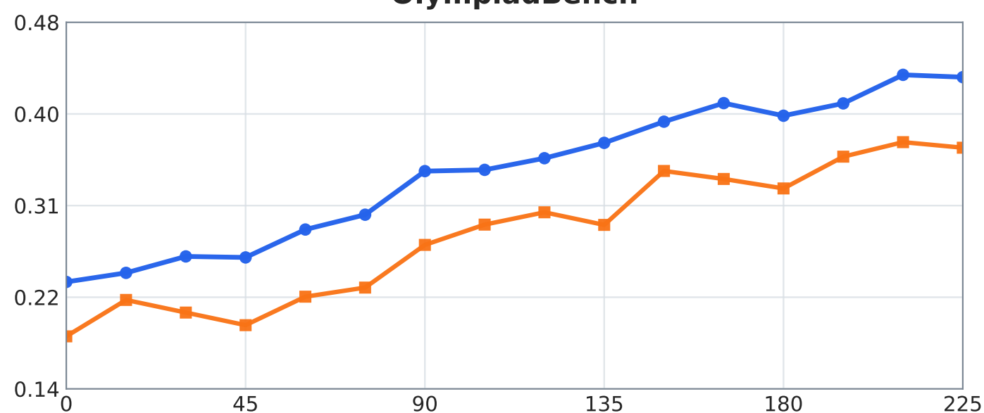
OlympiadBench
