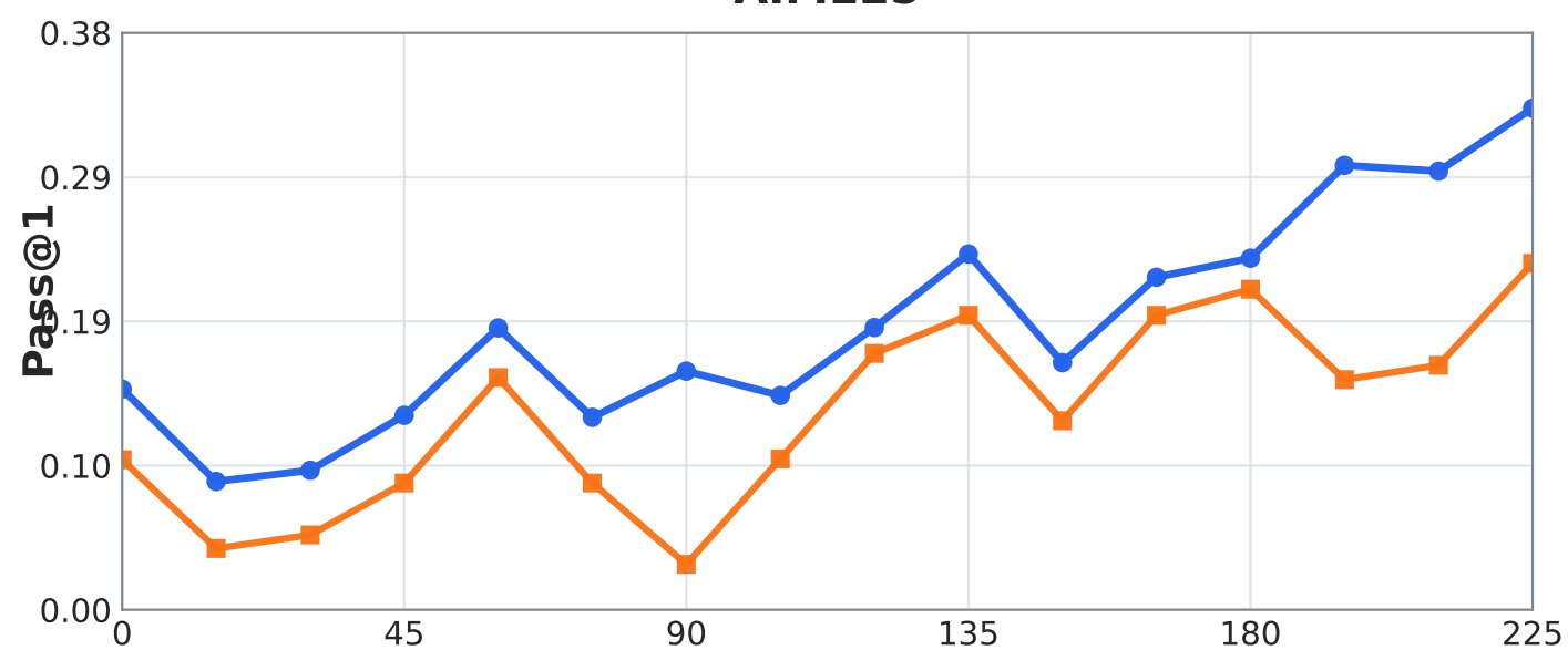
AIME25
