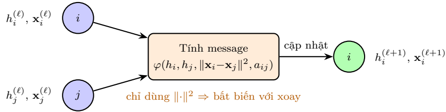
Hình 3.13: Cơ chế cập nhật tương biến: hàm message \varphi chỉ nhận khoảng cách bình phương \|\mathbf{x}_i - \mathbf{x}_j\|^2 (một đại lượng bất biến) thay vì tọa độ tuyệt đối, đảm bảo kết quả tương biến với nhóm E(3) .
