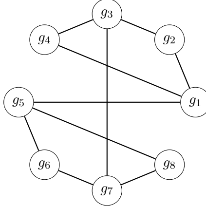
Hình 4.3: Minh họa đồ thị Cayley sinh bởi một tập con S .
