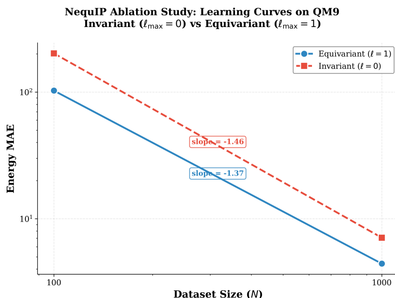
Hình 7.8: So sánh đường học của Baseline ( \ell_{\max} = 0 ) và NequIP ( \ell_{\max} = 1 ) trên hai kích thước tập dữ liệu.
