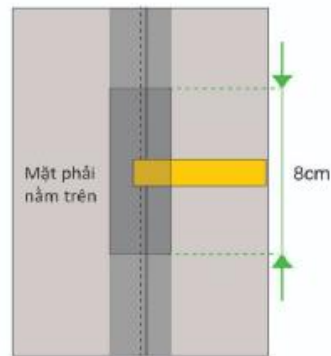
2 Ép seam lần 1
