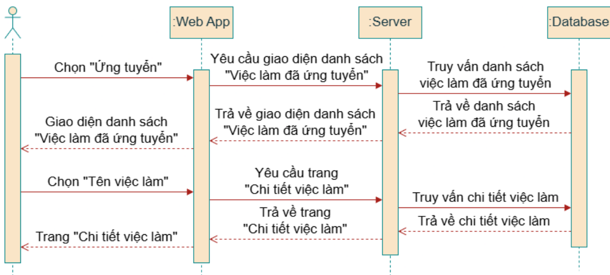
Hình 72. Sequence diagram 8 – Xem việc làm đã ứng tuyển
