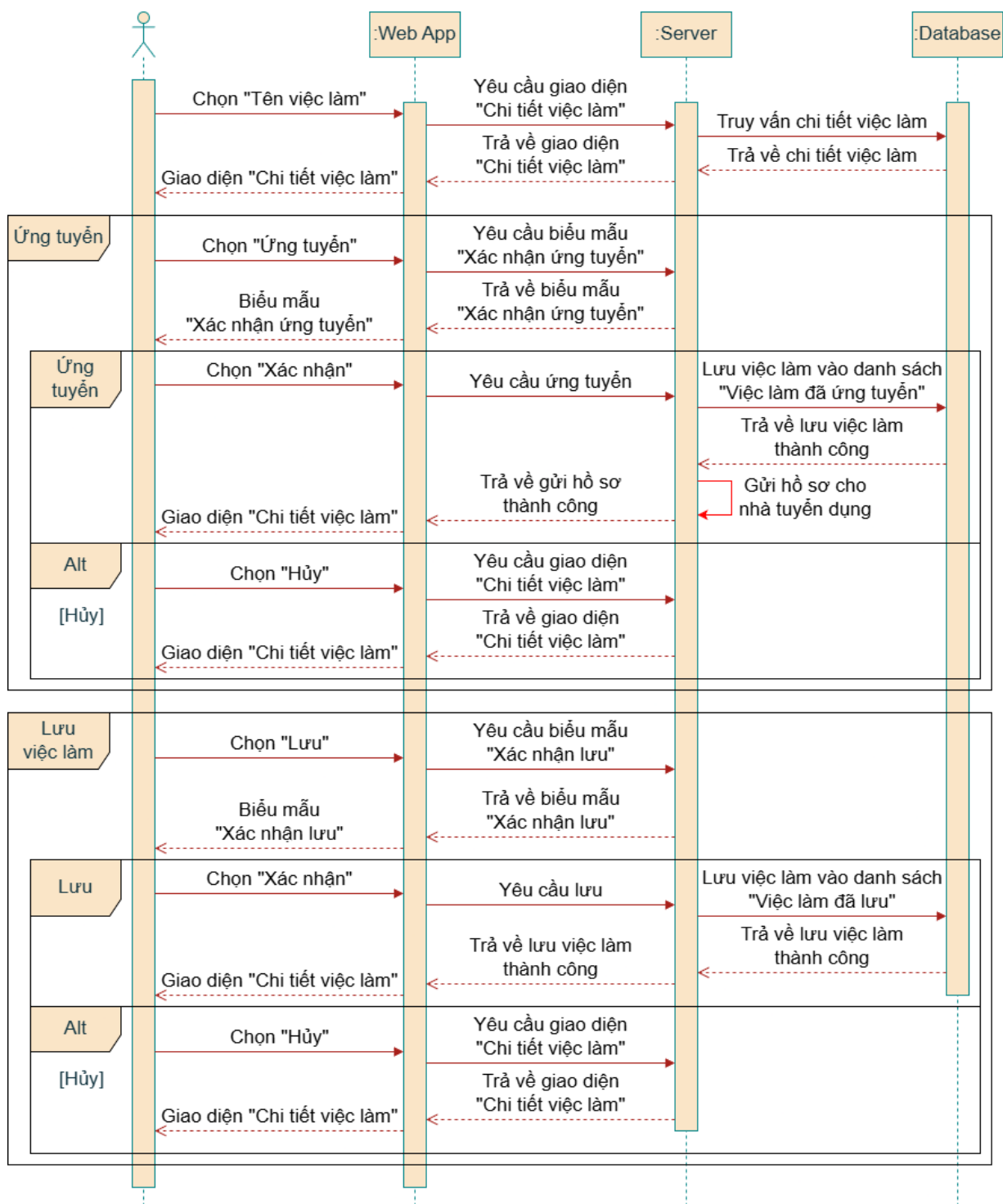
Hình 22: Sequence diagram 7 – Xem việc làm
