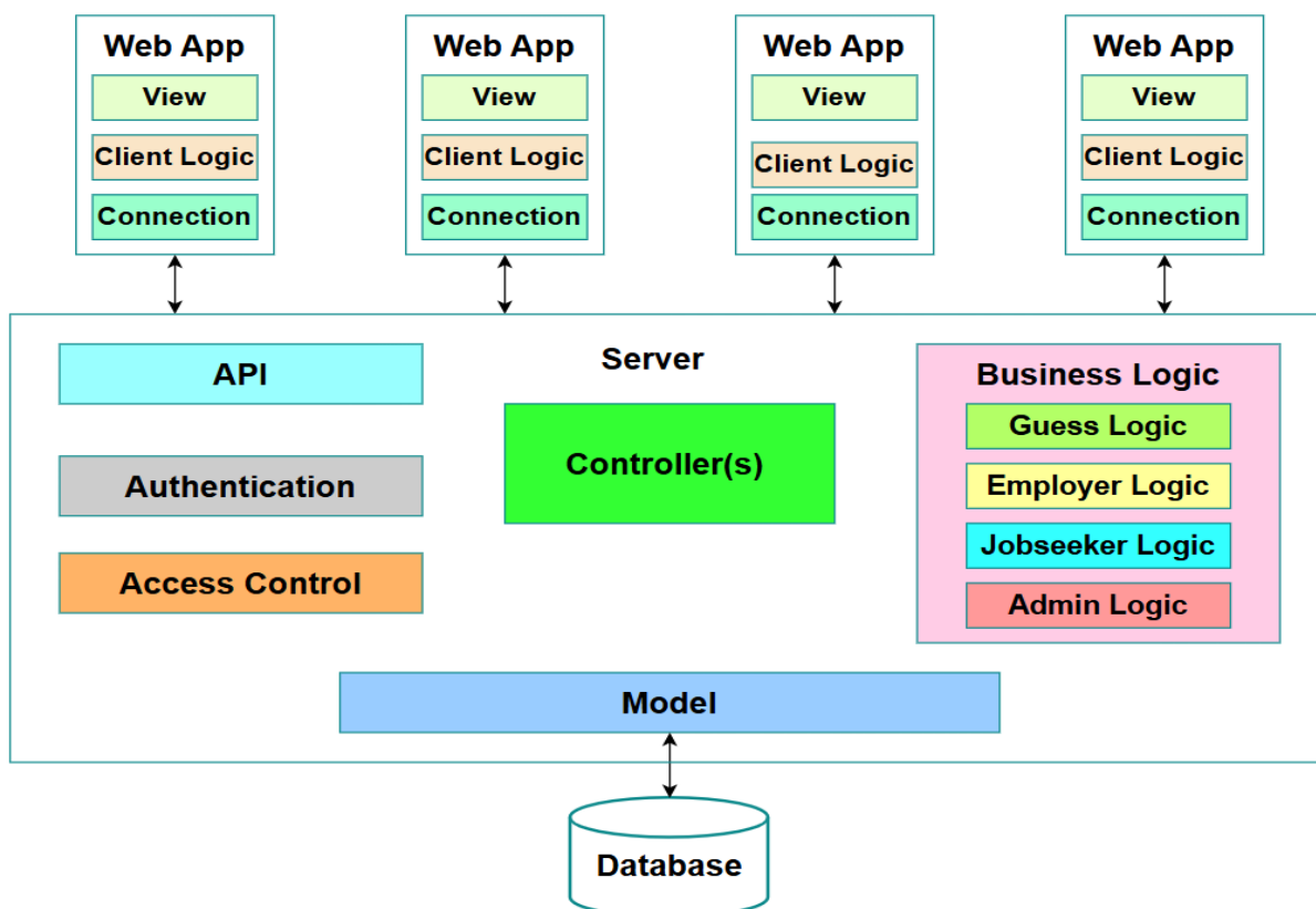
Hình 24: Kiến trúc cho toàn hệ thống
