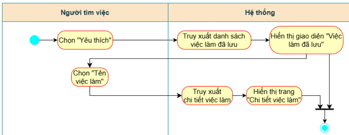
Hình 71. Activity diagram 9 - Xem việc làm đã lưu
