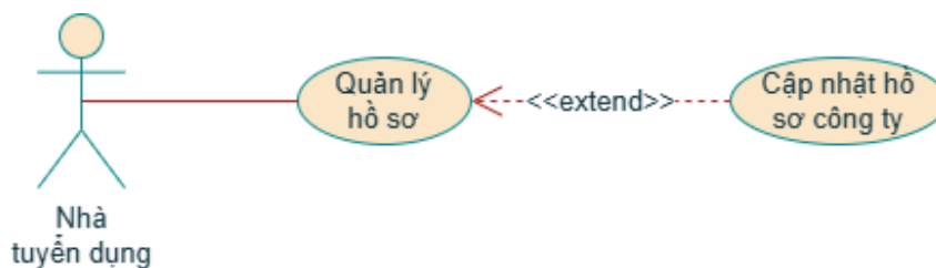
Hình 5: Use-case diagram 4 – Quản lý hồ sơ
