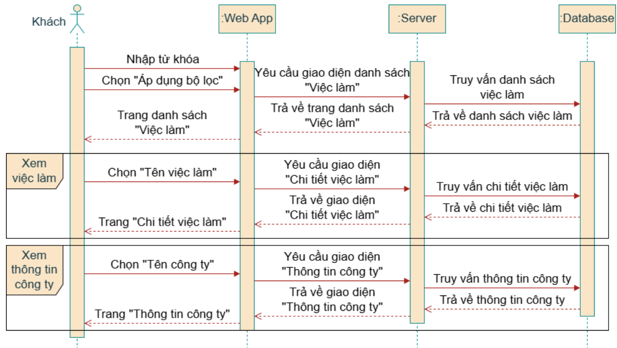
Hình 16: Sequence diagram 1 – Tìm việc làm
