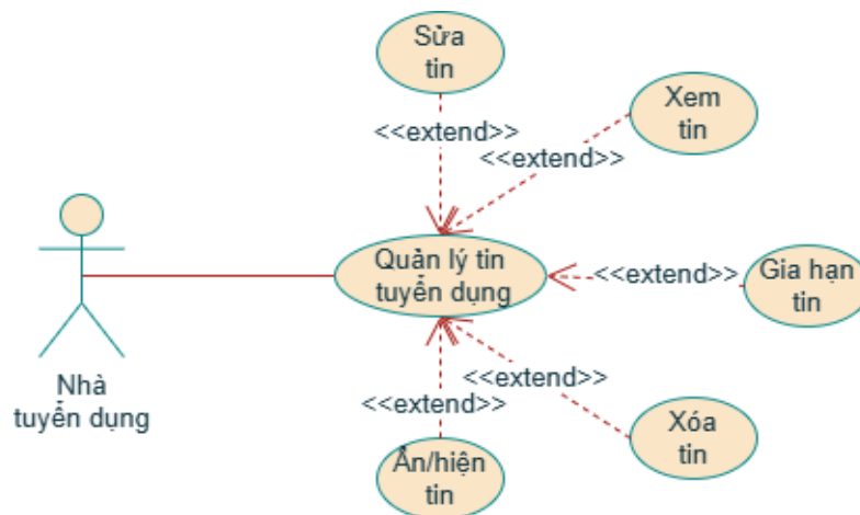
Hình 4: Use-case diagram 3 – Quản lý tin tuyển dụng
