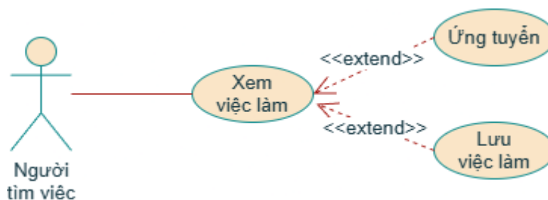
Hình 8: Use-case diagram 7 – Xem việc làm
