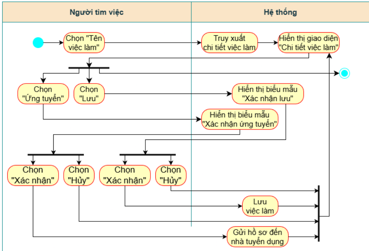
Hình 15: Activity diagram 7 – Xem việc làm
