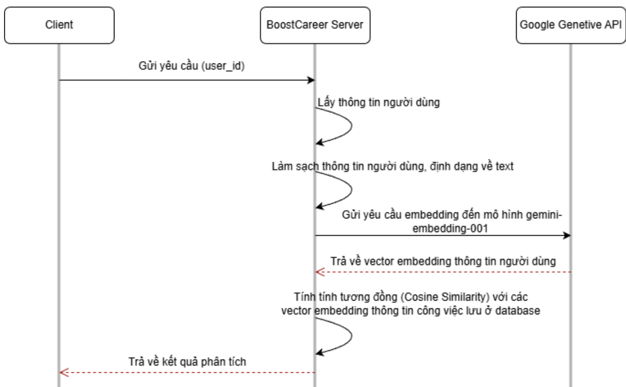
Hình 60. Mô hình ý tưởng tính năng gợi ý công việc phù hợp
