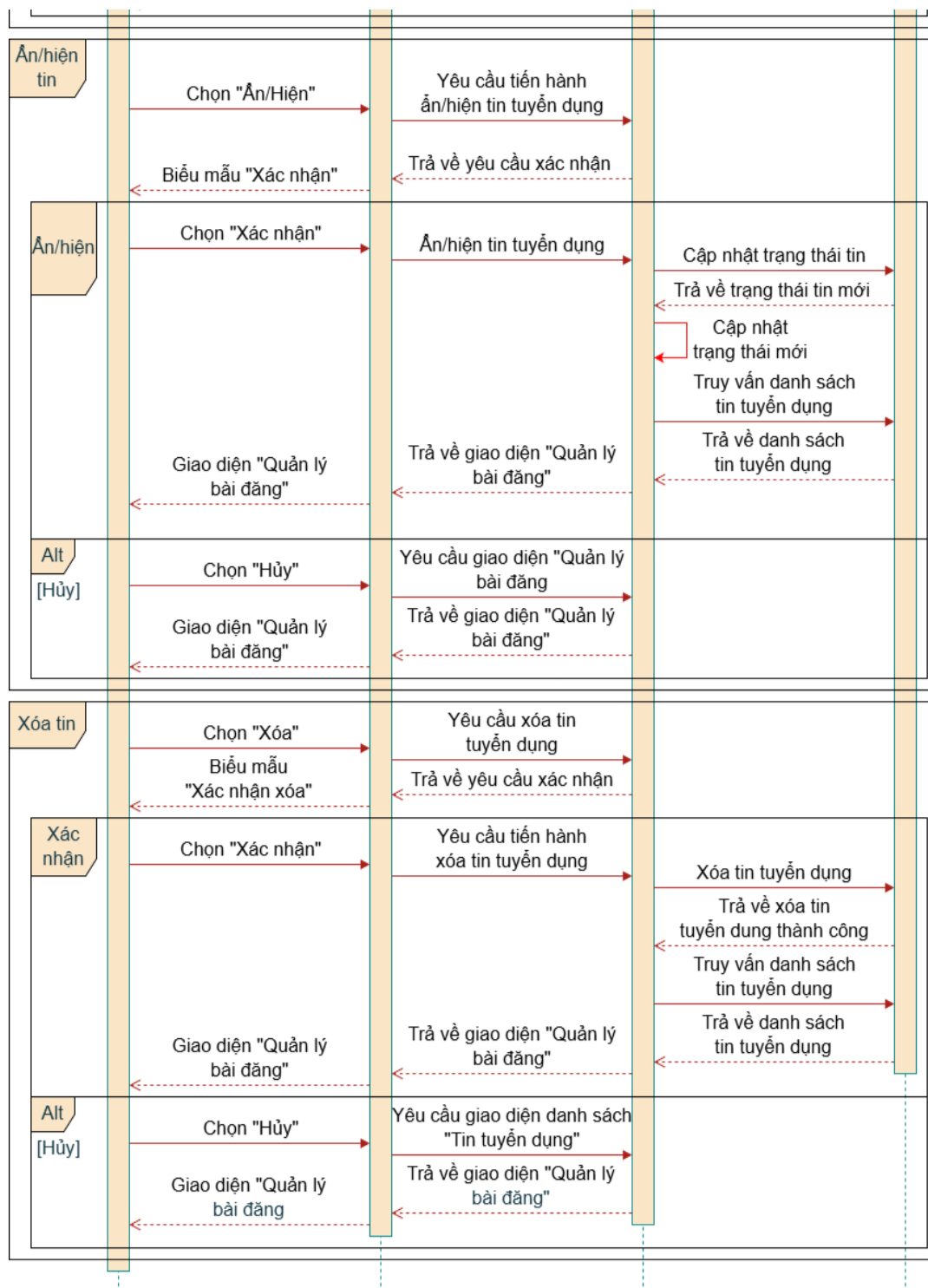
Hình 18: Sequence diagram 3 – Quản lý tin tuyển dụng
