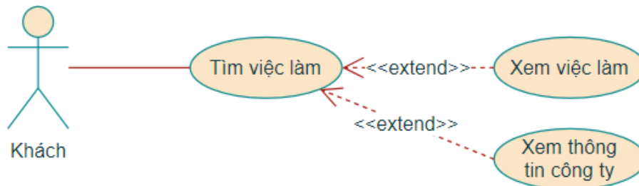
Hình 2: Use-case diagram 1 – Tìm việc làm
