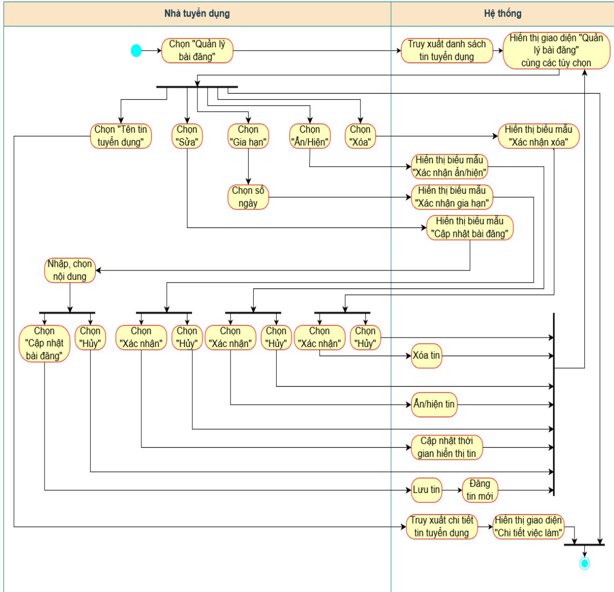
Hình 11: Activity diagram 3 – Quản lý tin tuyển dụng
