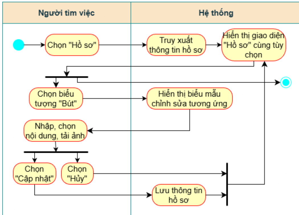
Hình 14: Activity diagram 6 – Xem hồ sơ cá nhân
