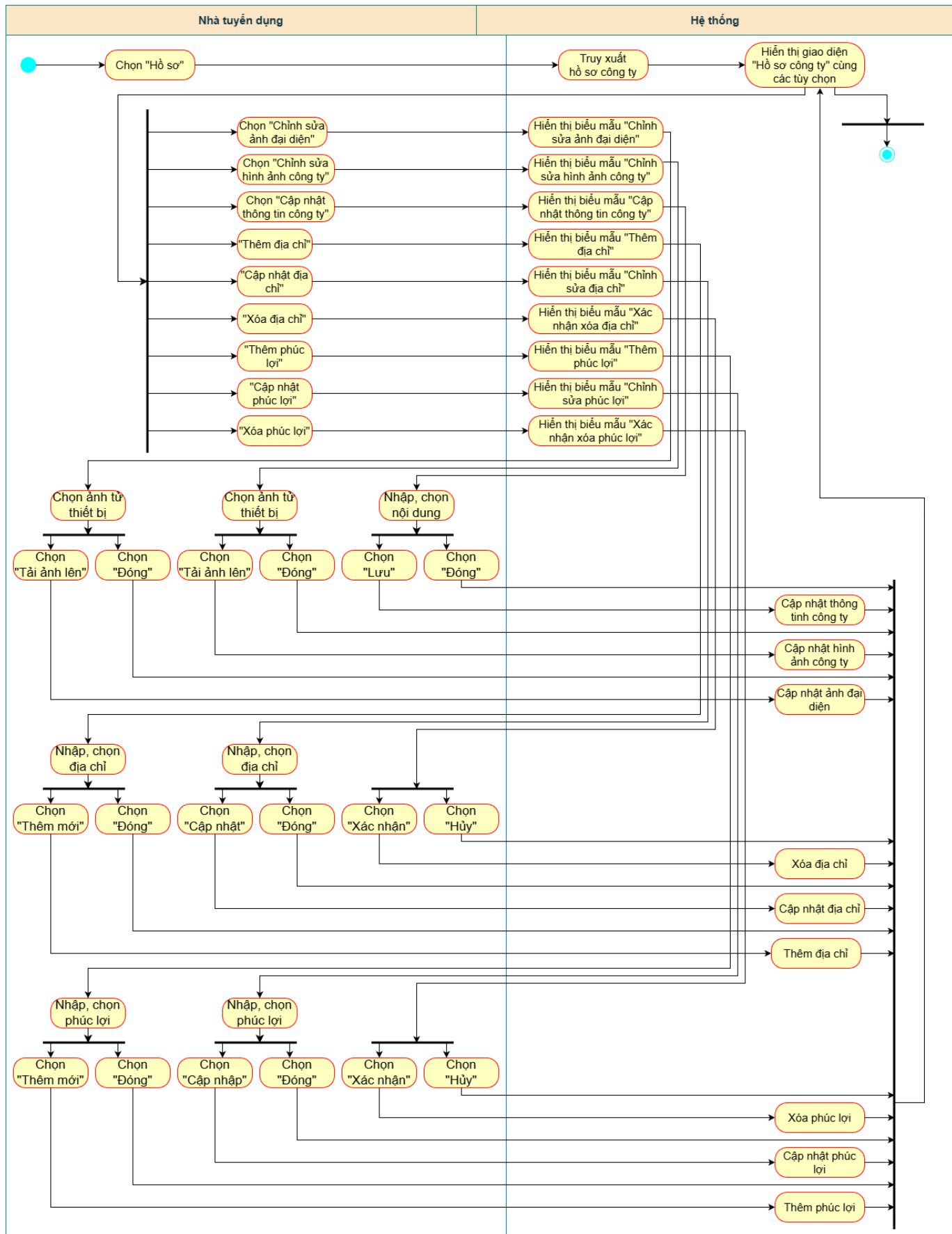
Hình 12: Activity diagram 4 – Quản lý hồ sơ
