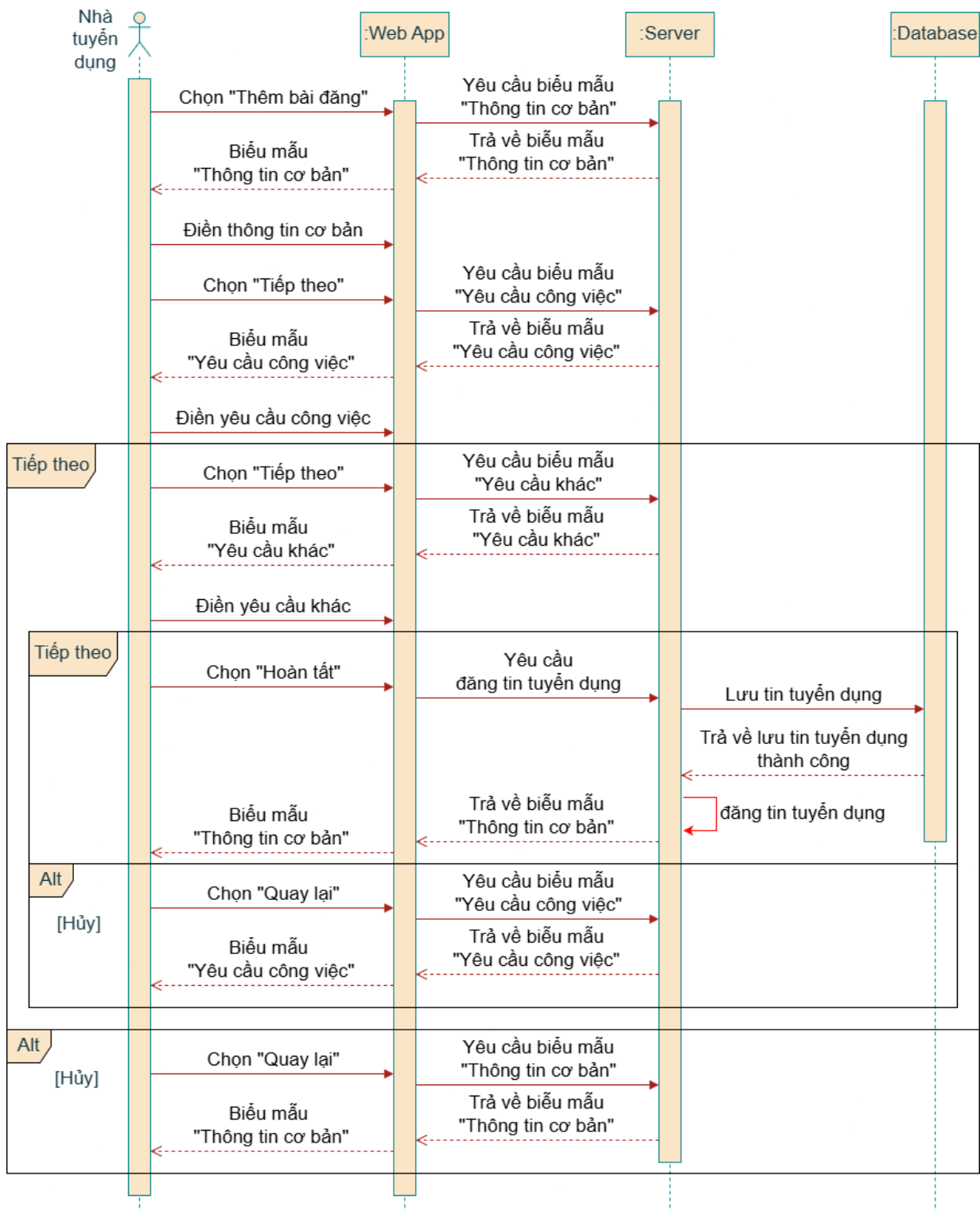
Hình 17. Sequence diagram 2 - Đăng tin tuyển dụng
