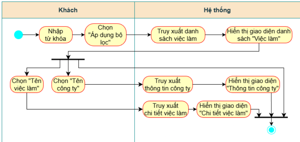
Hình 9: Activity diagram 1 – Tìm việc làm
