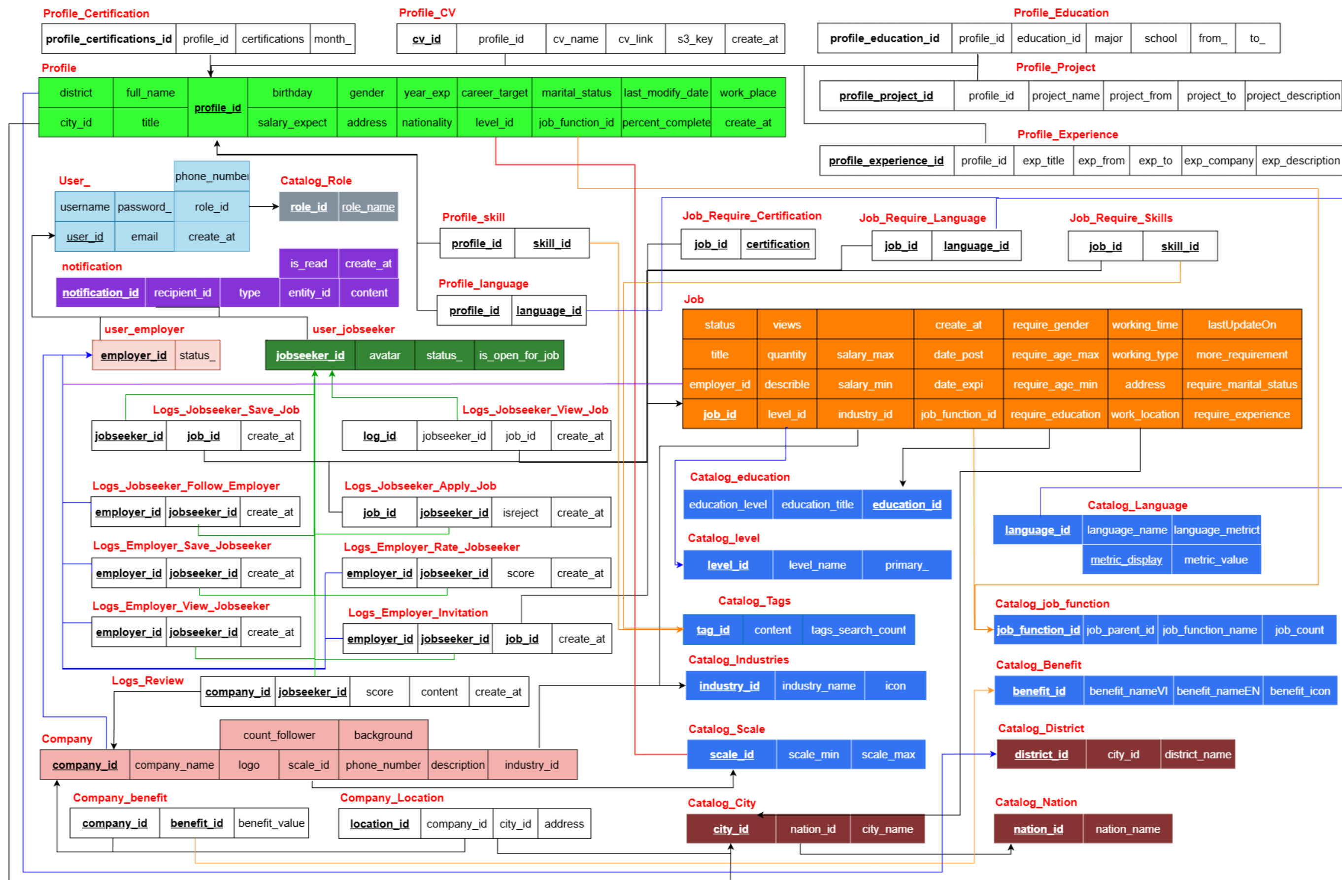
Hình 26: Relational data model
