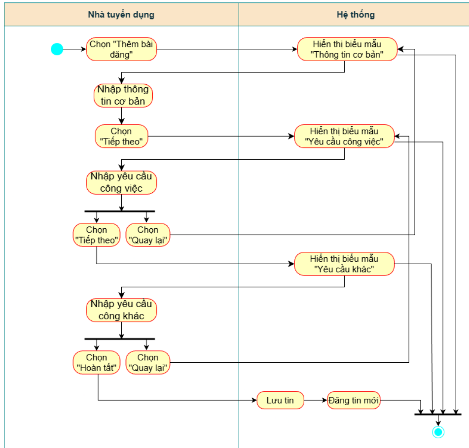
Hình 10. Activity diagram 2 - Đăng tin tuyển dụng
