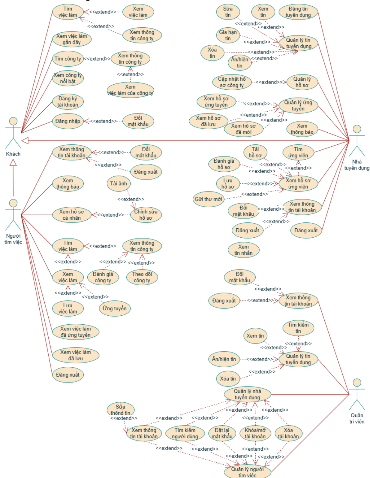
Hình 1: Use-case diagram toàn hệ thống
