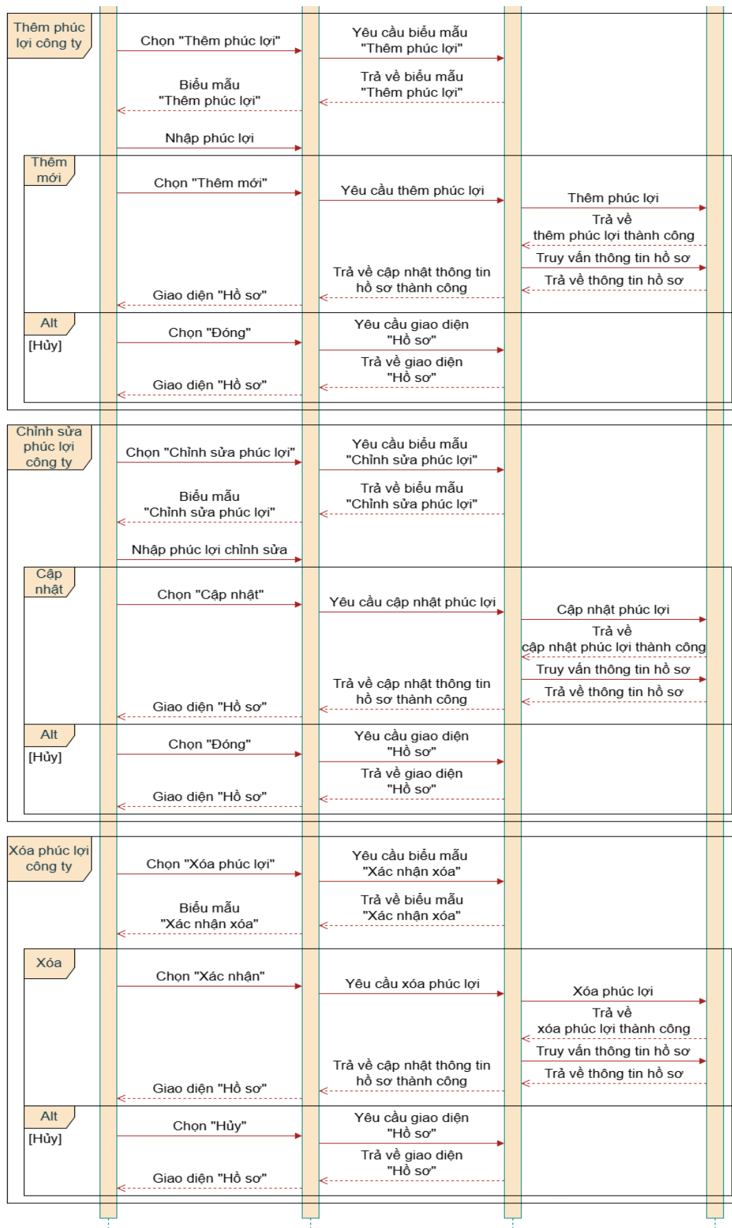
Hình 19: Sequence diagram 4 – Quản lý hồ sơ
