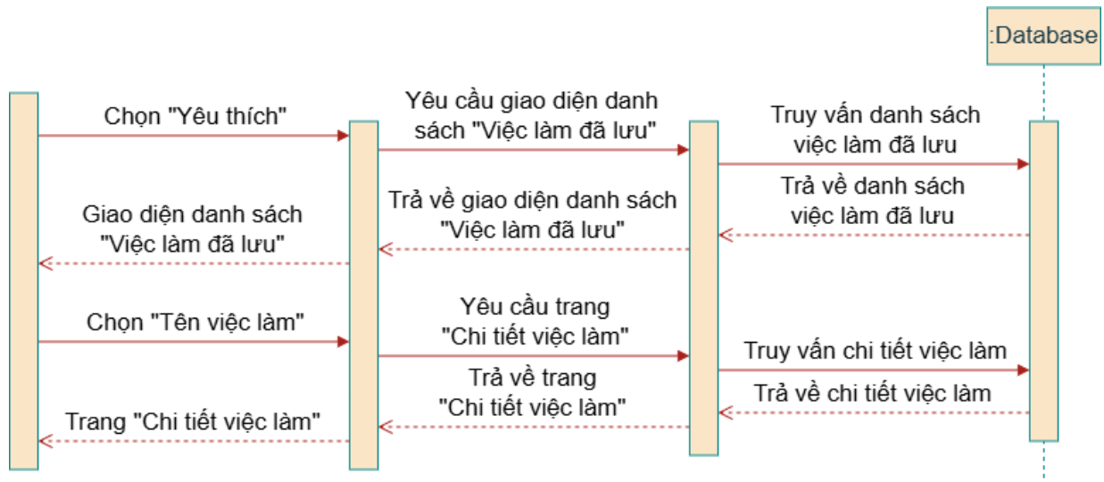
Hình 73. Sequence diagram 9 - Xem việc làm đã lưu
