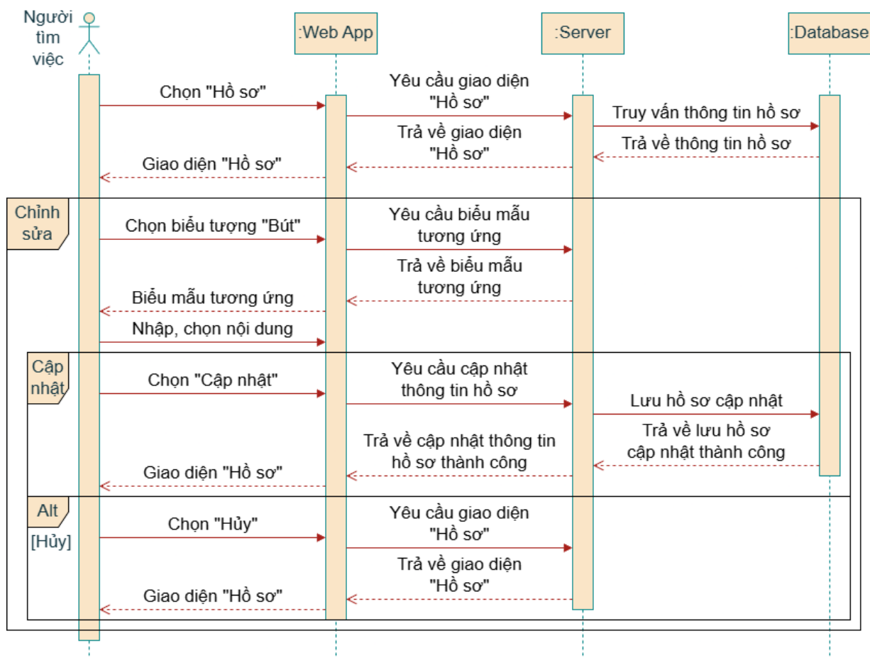
Hình 21: Sequence diagram 6 – Xem hồ sơ cá nhân
