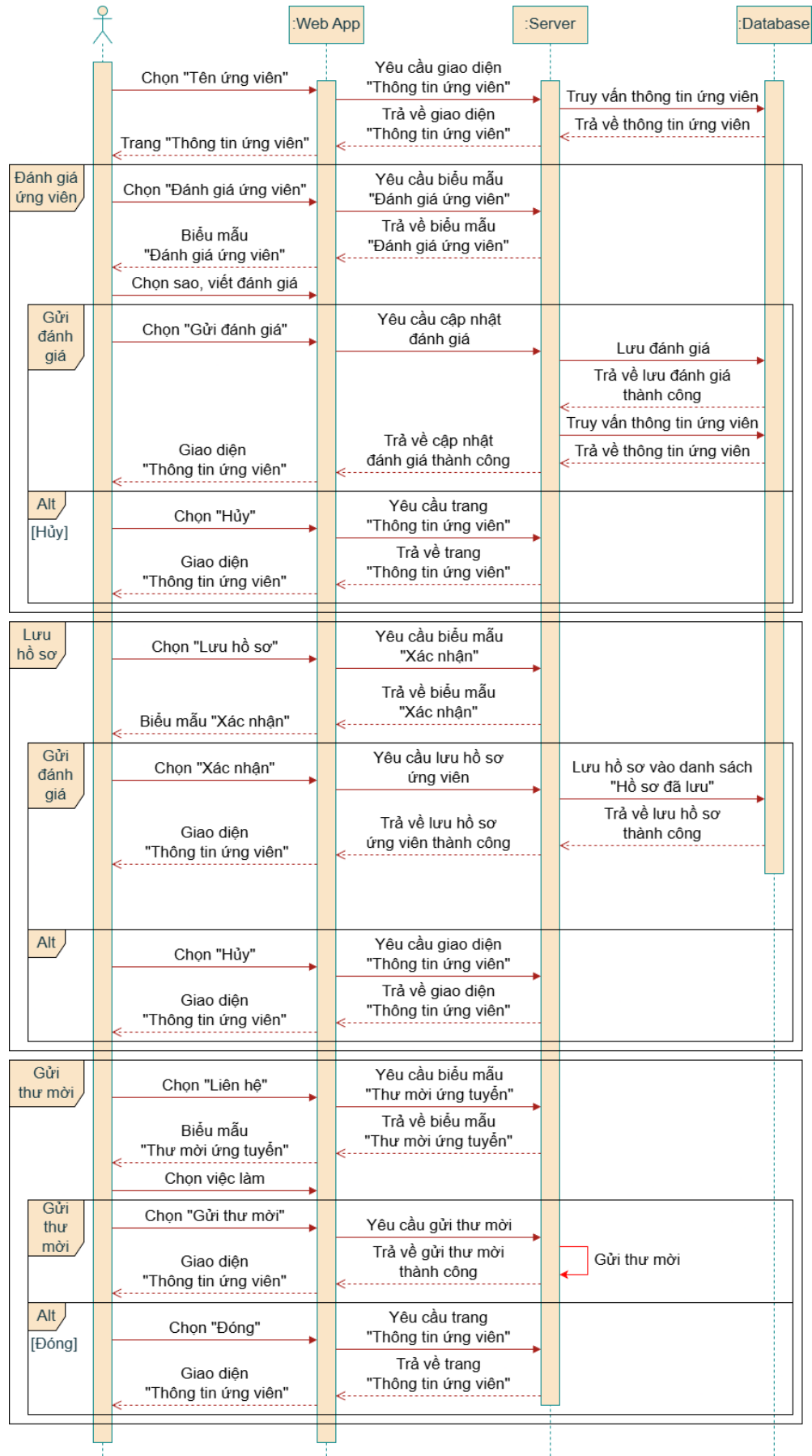
Hình 20: Sequence diagram 5 – Xem hồ sơ ứng viên
