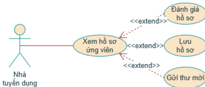
Hình 6: Use-case diagram 5 – Xem hồ sơ ứng viên
