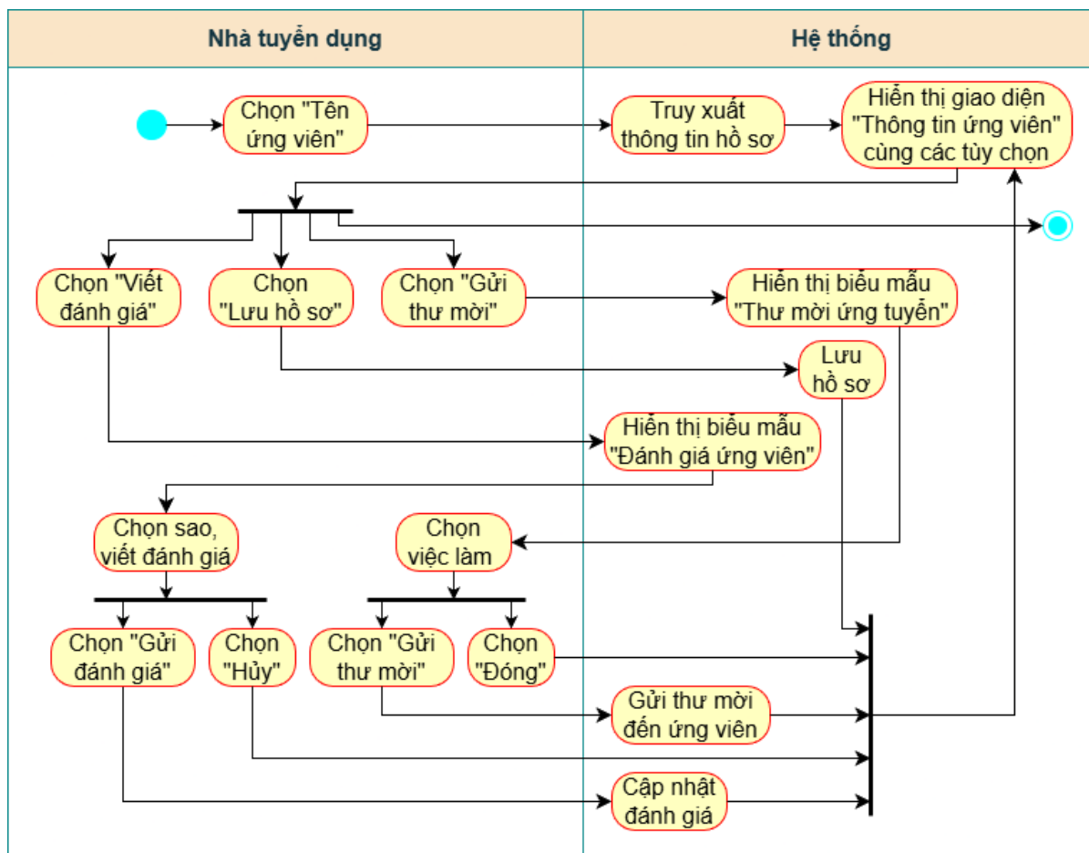
Hình 13: Activity diagram 5 – Xem hồ sơ ứng viên
