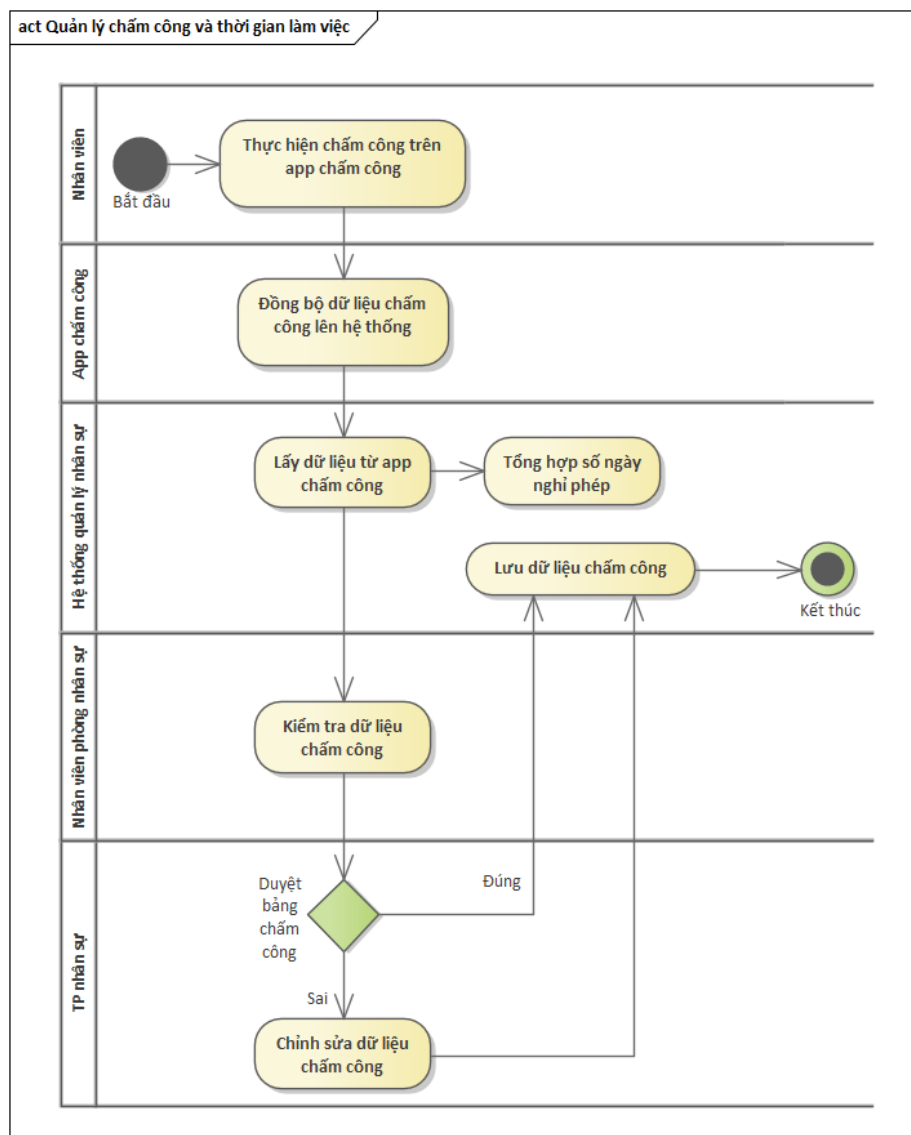
Hình 3. 6: Sơ đồ quy trình nghiệp vụ quản lý chấm công - nghỉ phép
