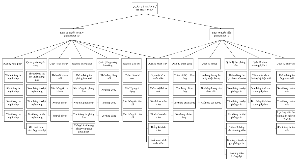
Hình 3. 13: Sơ đồ phân rã chức năng hệ thống quản lý nhân sự TH True Milk
