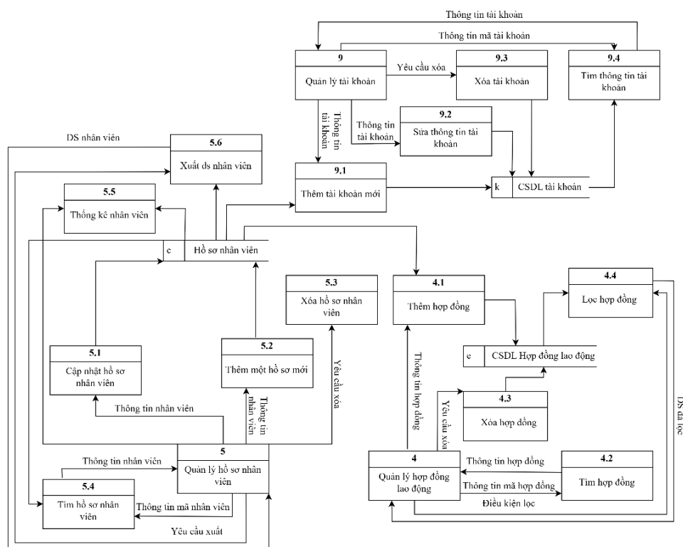
Hình 3. 17: Sơ đồ dòng dữ liệu mức 2 quản lý hồ sơ nhân viên
