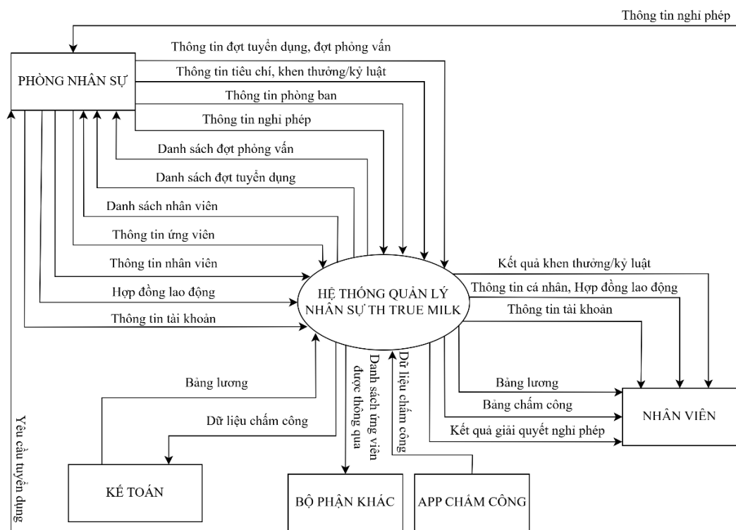
Hình 3. 14: Sơ đồ dòng dữ liệu mức 0
