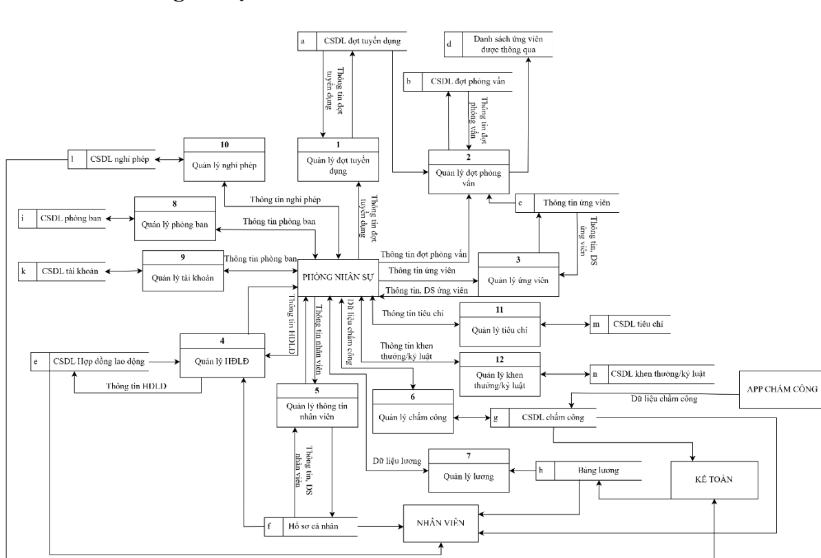
Hình 3. 15: Sơ đồ dòng dữ liệu mức 1
