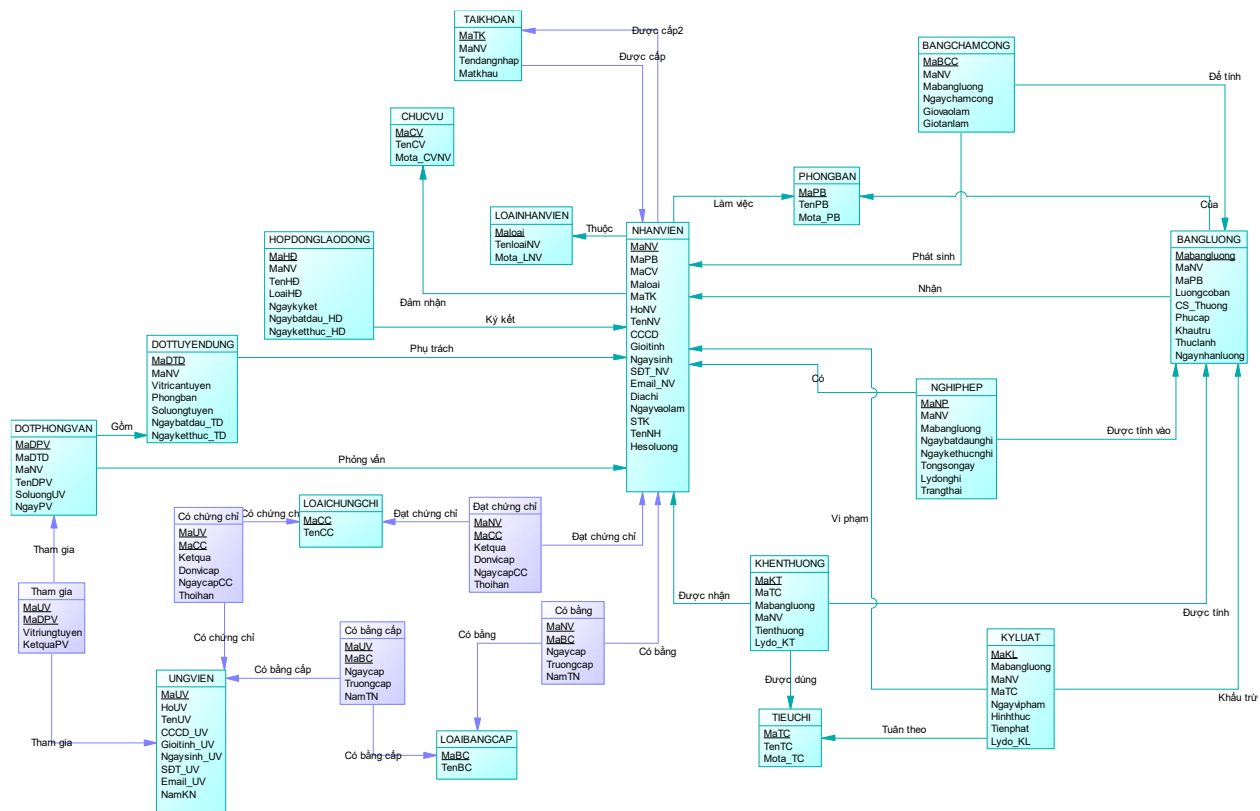
Hình 3. 11: Sơ đồ cơ sở dữ liệu mức vật lý của hệ thống
