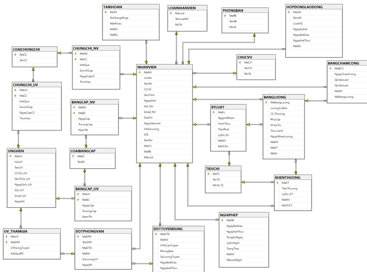
Hình 3. 12: Cấu trúc Diagram hệ thống
