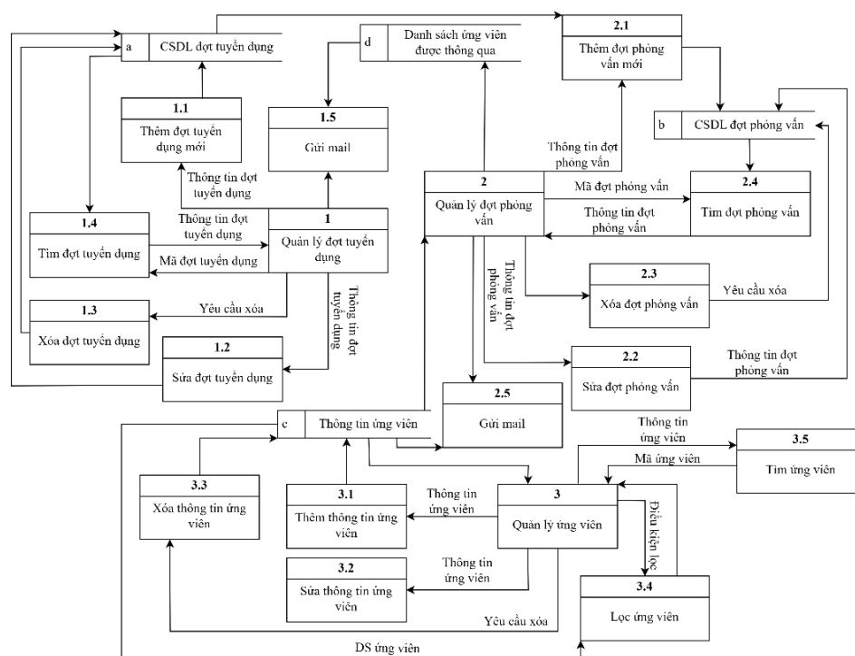
Hình 3. 16: Sơ đồ dòng dữ liệu mức 2 quản lý tuyển dụng
