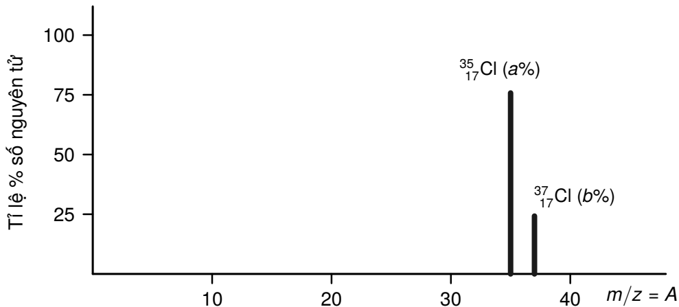
Hình 2.2. Phổ khối lượng của chlorine
