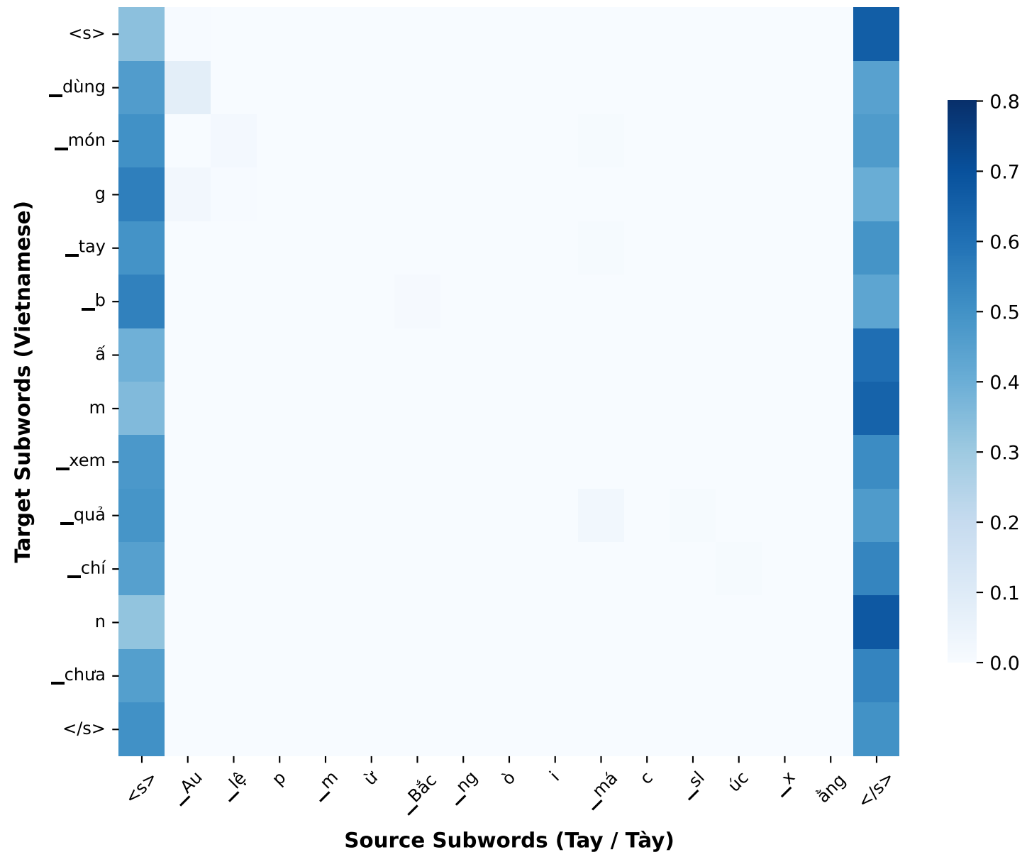
(b) TSSA (Ours)
